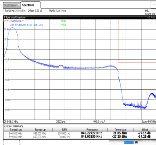
Band26(824-849)-3MHz-QPSK-27025-1RB#0-PASS
