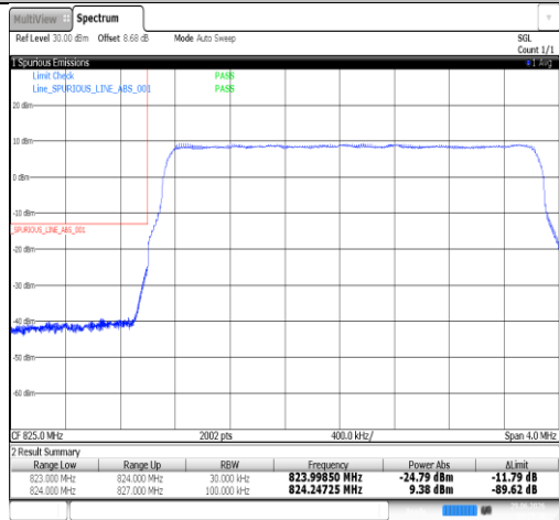
Band26(824-849)-3MHz-QPSK-26805-15RB#0-PASS
