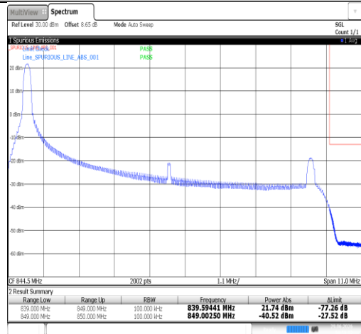
Band26(824-849)-10MHz-QPSK-26990-1RB#0-PASS
