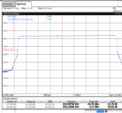
Band26(824-849)-10MHz-QPSK-26840-50RB#0-PASS
