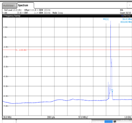
Band26(824-849)-10MHz-QPSK-26990-1RB#0-30~1000-PASS
