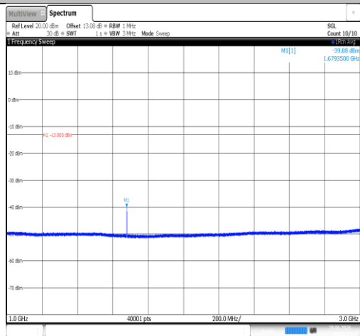
Band26(824-849)-10MHz-16QAM-26990-1RB#0- 1000~3000-PASS
