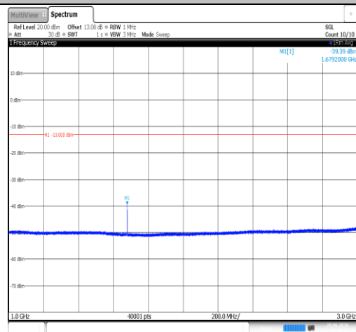
Band26(824-849)-10MHz-QPSK-26990-1RB#0-1000~3000-PASS
