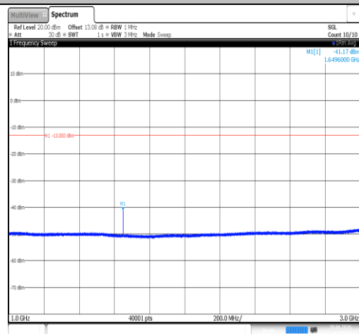
Band26(824-849)-15MHz-QPSK-26865-1RB#0- 1000~3000-PASS
