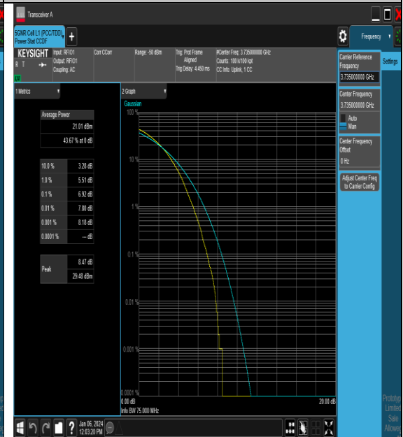
NTNV_N77-3700-3980_PC2_30_70_L_TID5_#1
