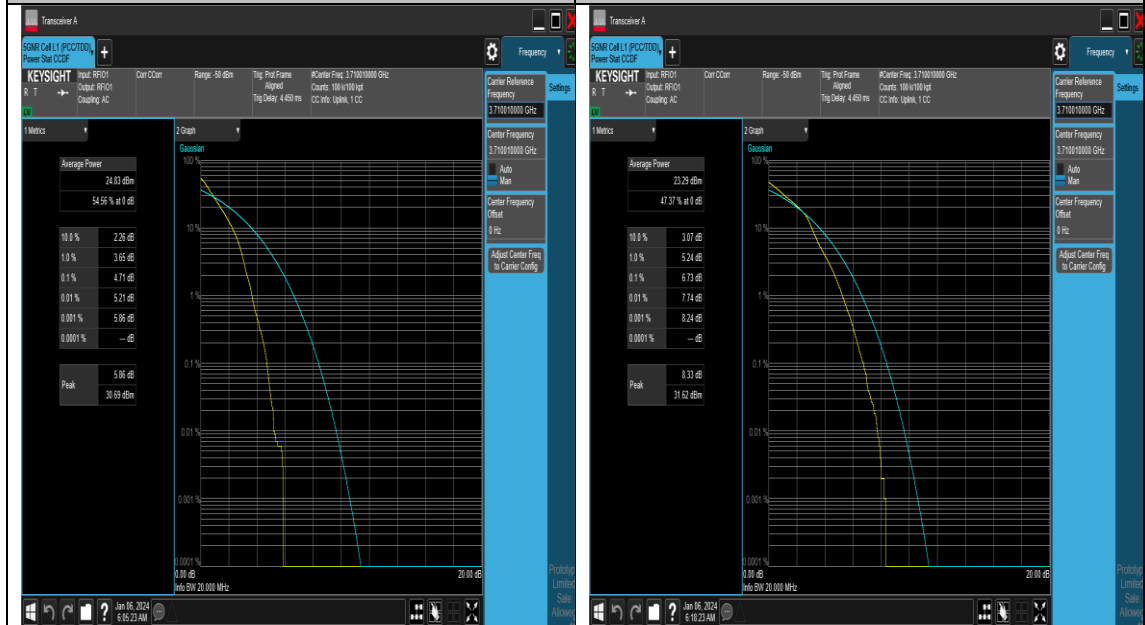
NTNV_N77-3700-3980_PC2_30_20_L_TID1_#1
