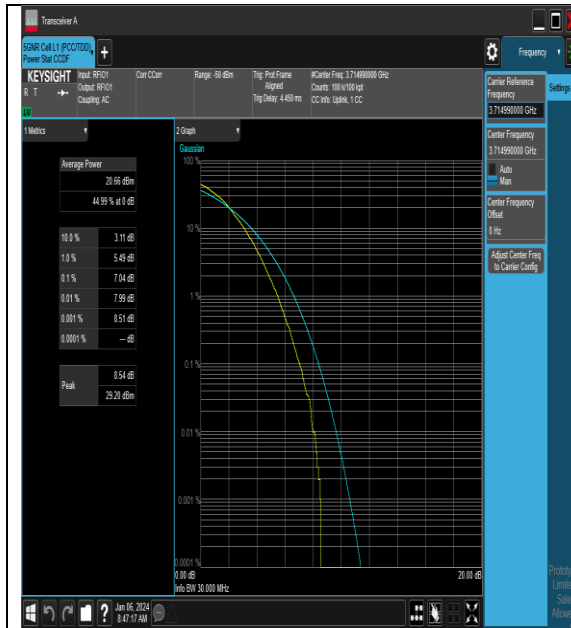
NTNV_N77-3700-3980_PC2_30_30_L_TID5_#1
