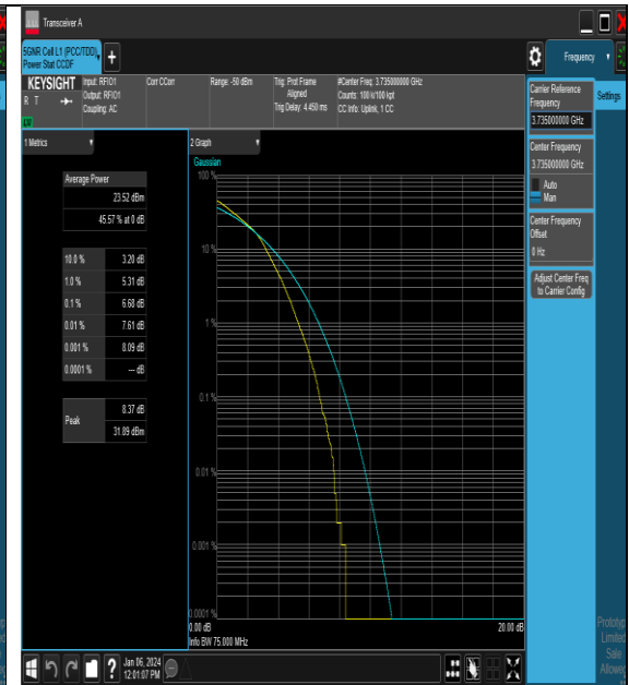
NTNV_N77-3700-3980_PC2_30_70_L_TID3_#1
