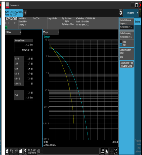
NTNV_N77-3700-3980_PC2_30_60_L_TID2_#1
