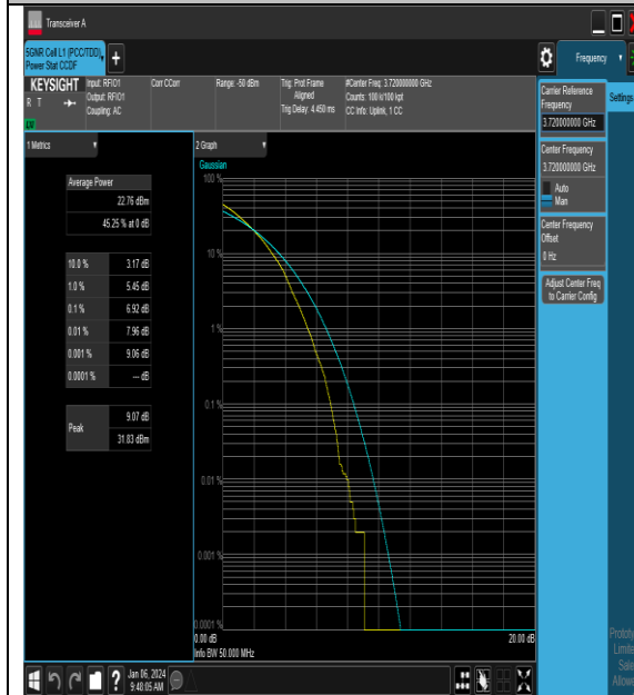
NTNV_N77-3700-3980_PC2_30_40_L_TID4_#1
