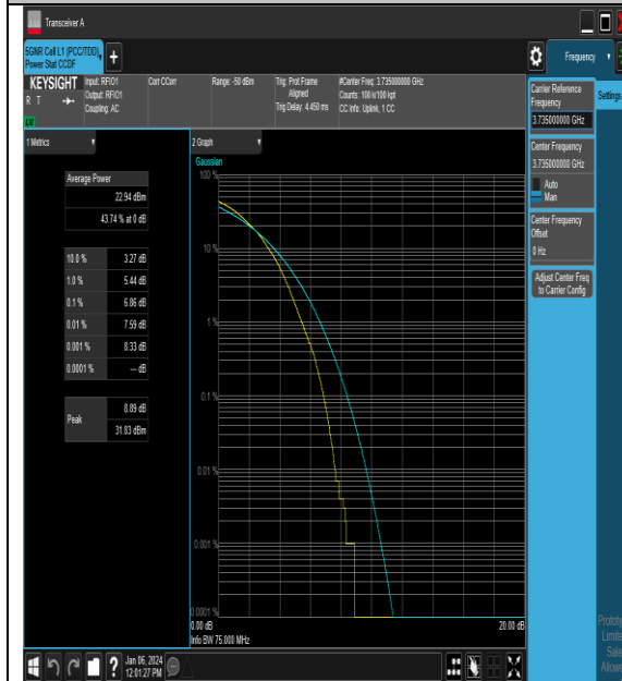
NTNV_N77-3700-3980_PC2_30_70_L_TID4_#1
