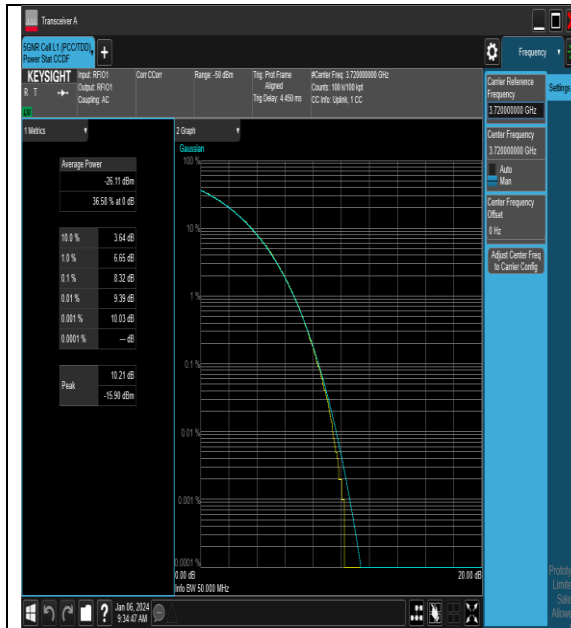
NTNV_N77-3700-3980_PC2_30_40_L_TID1_#1
