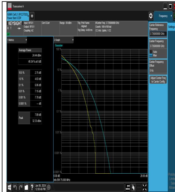
NTNV_N77-3700-3980_PC2_30_70_L_TID2_#1
