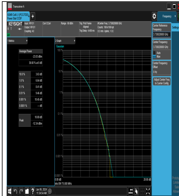
NTNV_N77-3700-3980_PC2_30_60_L_TID1_#1
