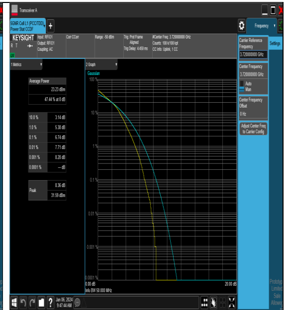
NTNV_N77-3700-3980_PC2_30_40_L_TID3_#1
