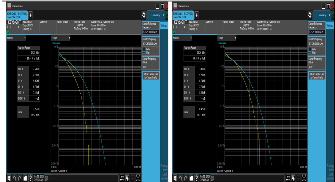
NTNV_N77-3700-3980_PC2_30_25_L_TID2_#1
