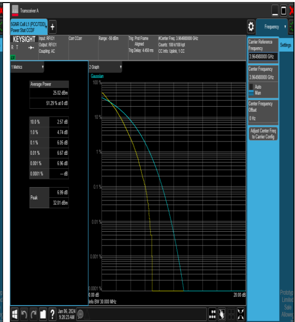
NTNV_N77-3700-3980_PC2_30_30_H_TID2_#1
