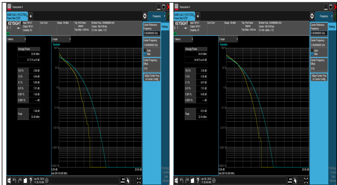
NTNV_N77-3700-3980_PC2_30_50_H_TID2_#1
