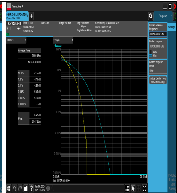
NTNV_N77-3700-3980_PC2_30_70_H_TID1_#1
