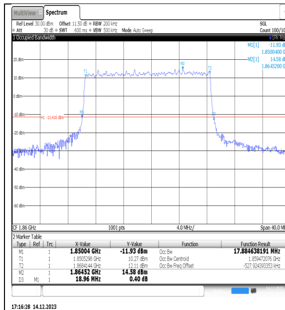
NTNV_N25_PC3_15_20_L_TID1_Ant1#1
