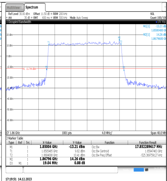
NTNV_N25_PC3_15_20_L_TID2_Ant1#1
