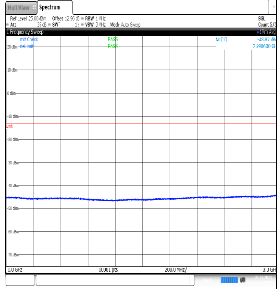
NTNV_N77-3450- 3550_PC2_30_70_L_TID2_NS_01_0.15_30_#1
