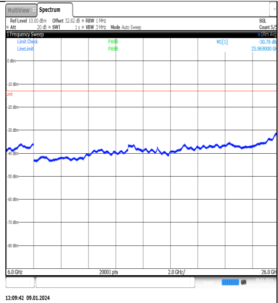
NTNV_N77-3700- 3980_PC2_30_70_L_TID13_NS_01_6000_26000 _#1
