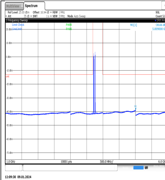
NTNV_N77-3700- 3980_PC2_30_70_L_TID13_NS_01_1000_6000_ _#1
