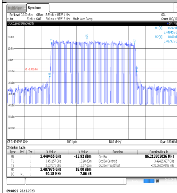
NTNV_N77-3450- 3550_PC2_30_90_L_TID3_Ant1#1
