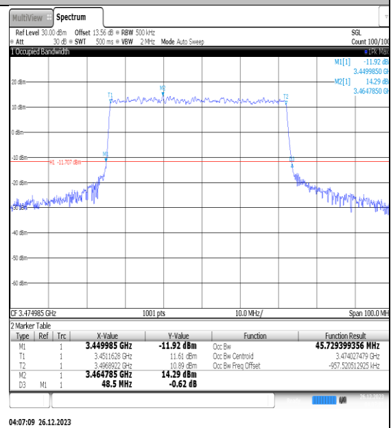
NTNV_N77-3450- 3550_PC2_30_50_L_TID4_Ant1#1
