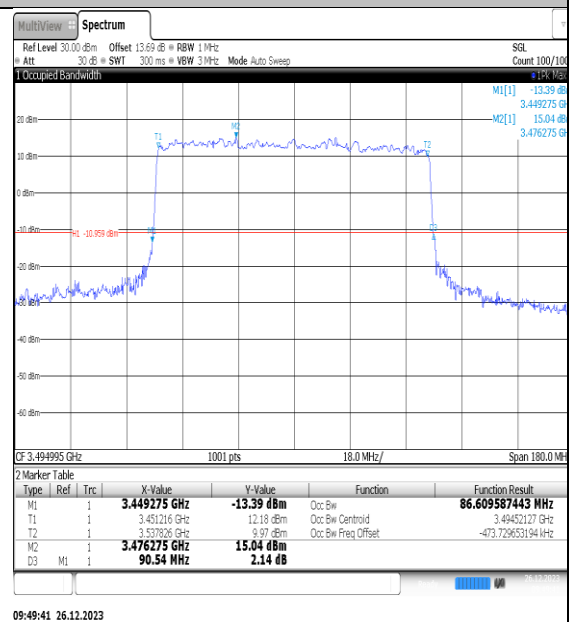
NTNV_N77-3450- 3550_PC2_30_90_L_TID4_Ant1#1
