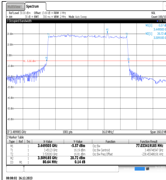
NTNV_N77-3450- 3550_PC2_30_80_L_TID1_Ant1#1
