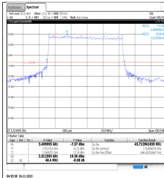
NTNV_N77-3450- 3550_PC2_30_50_H_TID1_Ant1#1
