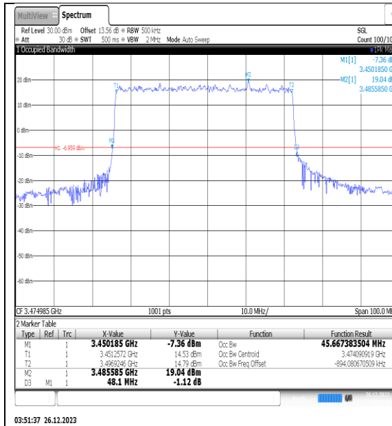
NTNV_N77-3450- 3550_PC2_30_50_L_TID1_Ant1#1
