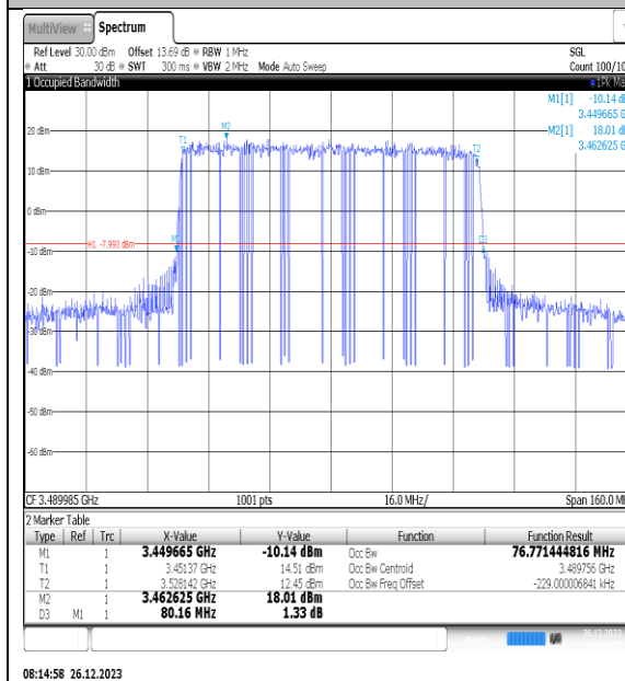
NTNV_N77-3450- 3550_PC2_30_80_L_TID3_Ant1#1
