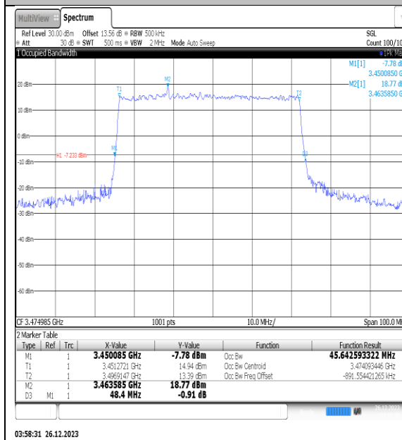
NTNV_N77-3450- 3550_PC2_30_50_L_TID3_Ant1#1
