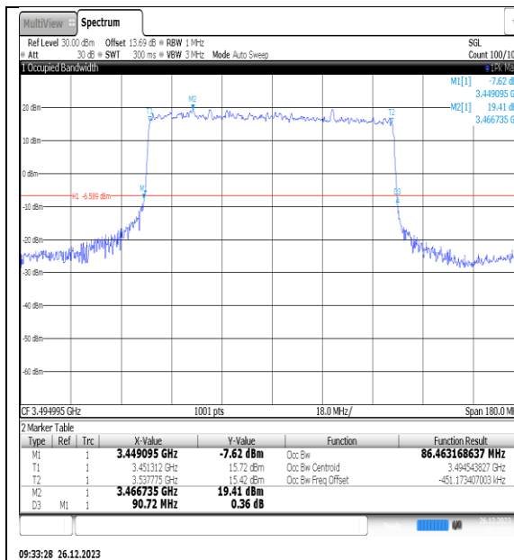
NTNV_N77-3450- 3550_PC2_30_90_L_TID1_Ant1#1
