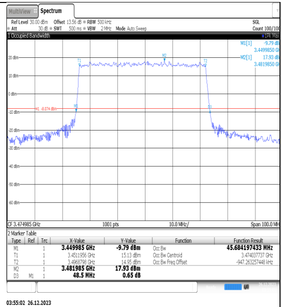
NTNV_N77-3450- 3550_PC2_30_50_L_TID2_Ant1#1
