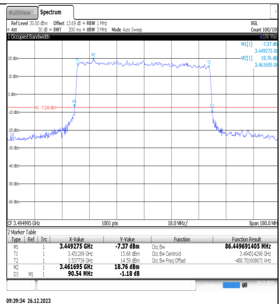
NTNV_N77-3450- 3550_PC2_30_90_L_TID2_Ant1#1
