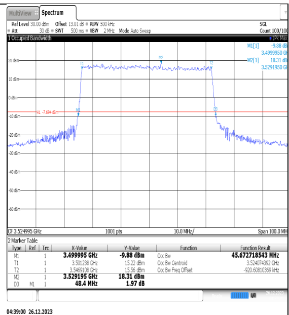
NTNV_N77-3450- 3550_PC2_30_50_H_TID2_Ant1#1
