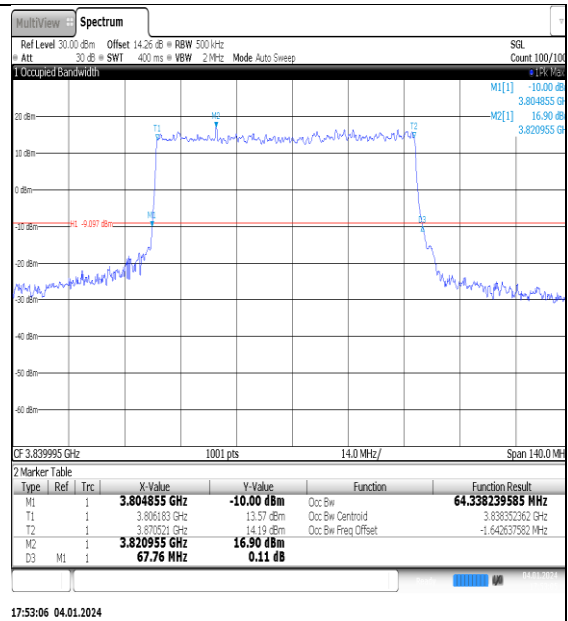
NTNV_N77-3700- 3980_PC2_30_70_M_TID2_Ant1#1
