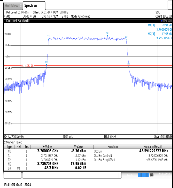
NTNV_N77-3700- 3980_PC2_30_50_L_TID1_Ant1#1
