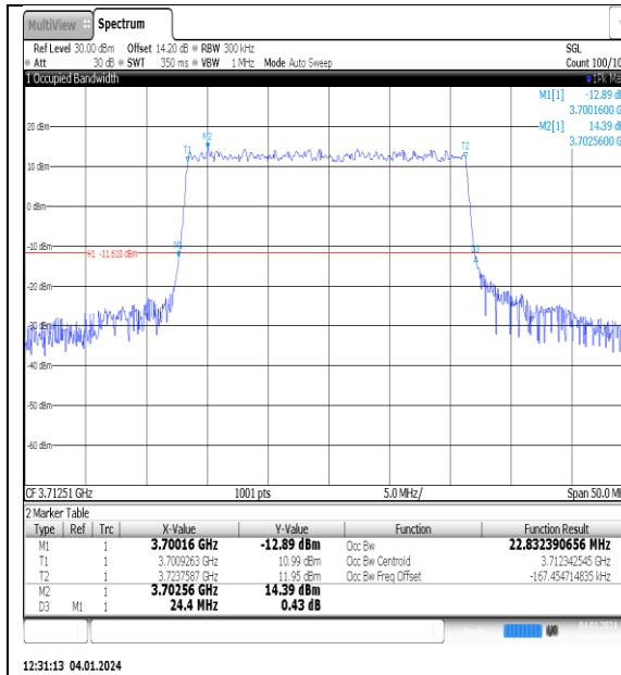
NTNV_N77-3700- 3980_PC2_30_25_L_TID4_Ant1#1
