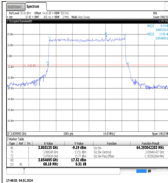
NTNV_N77-3700- 3980_PC2_30_70_M_TID1_Ant1#1
