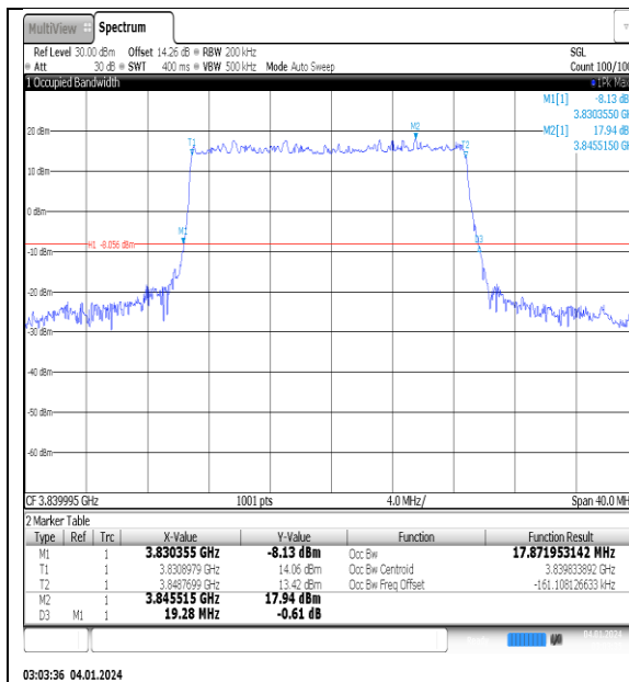
NTNV_N77-3700- 3980_PC2_30_20_M_TID1_Ant1#1
