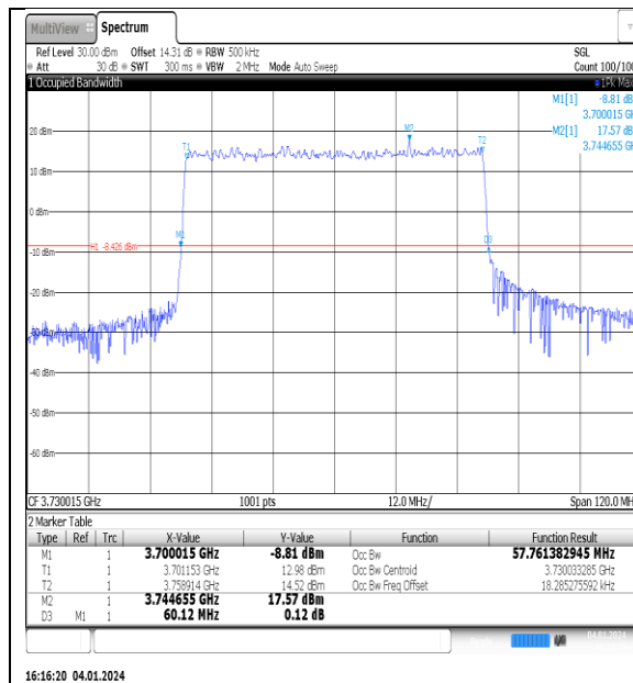
NTNV_N77-3700- 3980_PC2_30_60_L_TID1_Ant1#1
