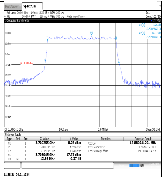
NTNV_N77-3700- 3980_PC2_30_15_L_TID4_Ant1#1
