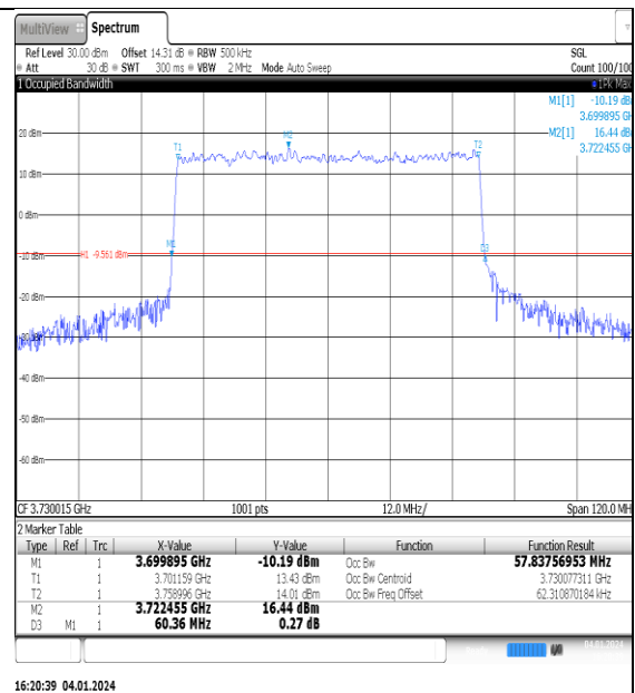
NTNV_N77-3700- 3980_PC2_30_60_L_TID2_Ant1#1
