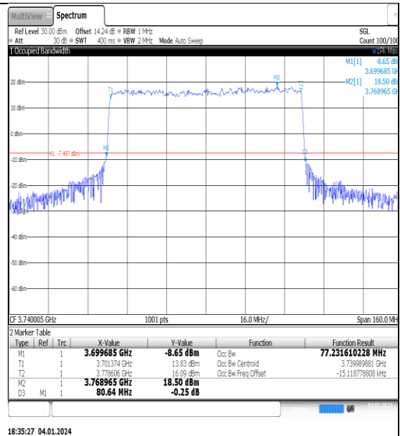
NTNV_N77-3700- 3980_PC2_30_80_L_TID2_Ant1#1
