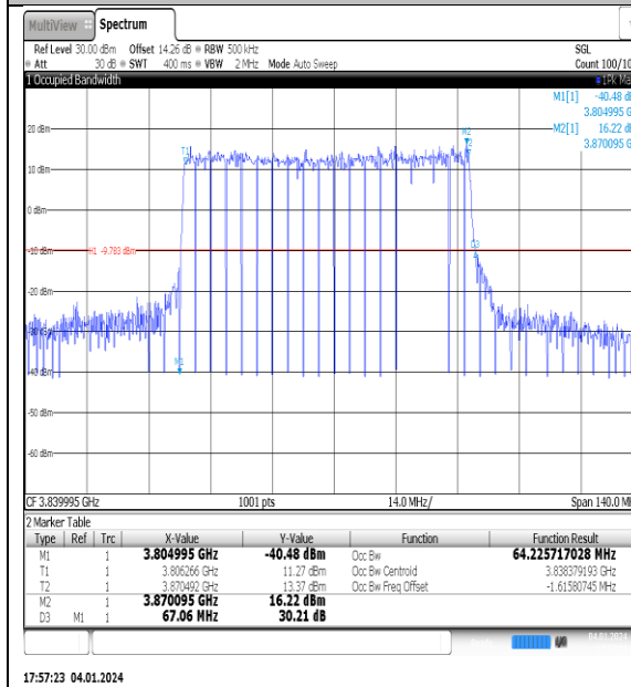
NTNV_N77-3700- 3980_PC2_30_70_M_TID3_Ant1#1
