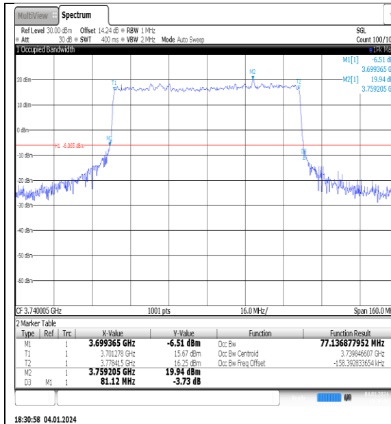
NTNV_N77-3700- 3980_PC2_30_80_L_TID1_Ant1#1
