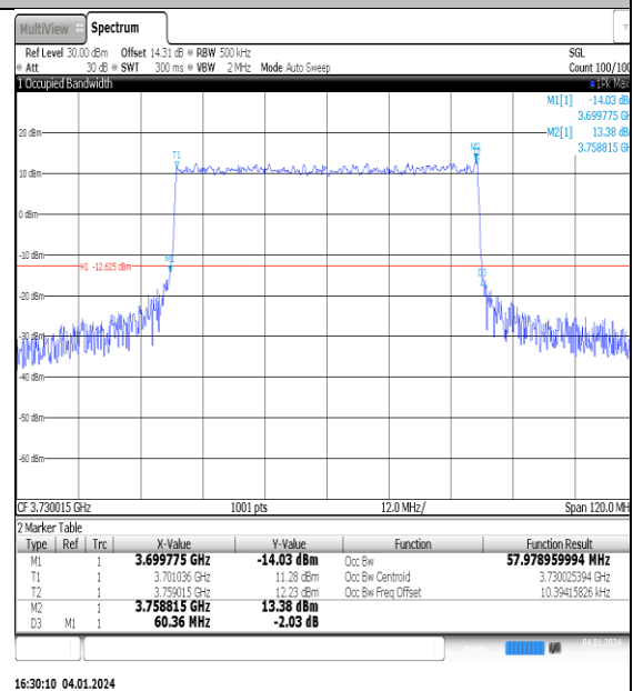
NTNV_N77-3700- 3980_PC2_30_60_L_TID4_Ant1#1
