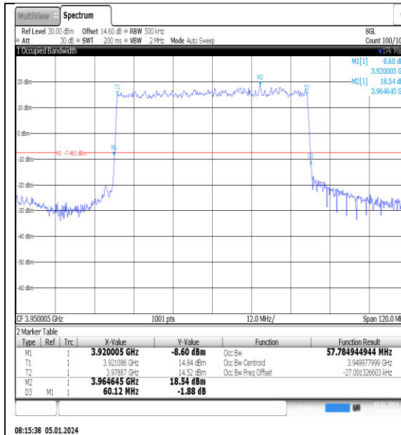
NTNV_N77-3700- 3980_PC2_30_60_H_TID1_Ant1#1
