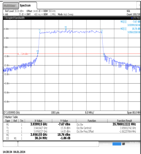
NTNV_N77-3700- 3980_PC2_30_40_H_TID3_Ant1#1
