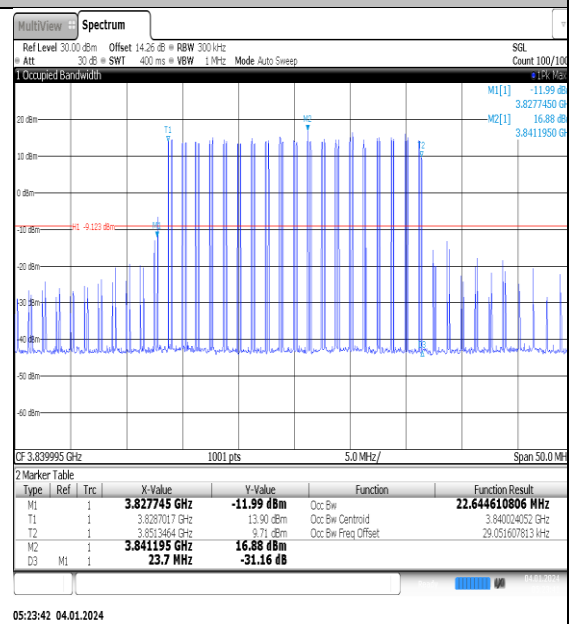
NTNV_N77-3700- 3980_PC2_30_25_M_TID3_Ant1#1
