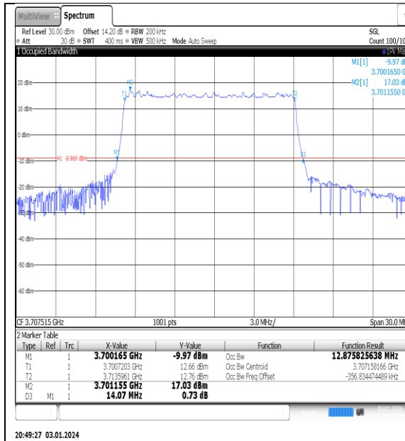
NTNV_N77-3700- 3980_PC2_30_15_L_TID3_Ant1#1
