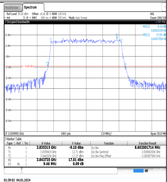
NTNV_N77-3700- 3980_PC2_30_10_M_TID2_Ant1#1
