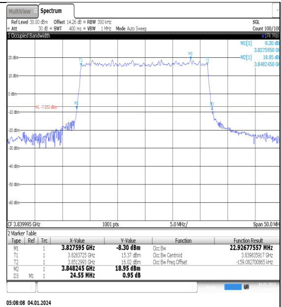
NTNV_N77-3700- 3980_PC2_30_25_M_TID1_Ant1#1
