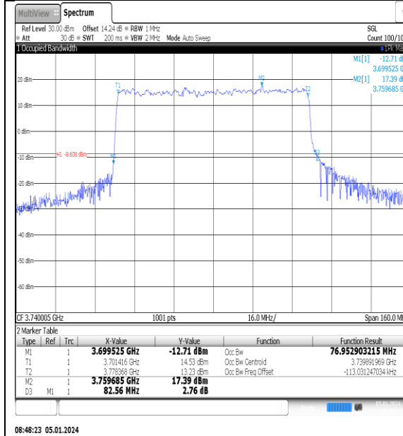
NTNV_N77-3700- 3980_PC2_30_80_L_TID3_Ant1#1
