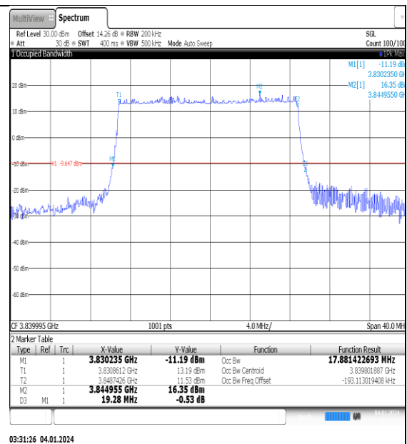
NTNV_N77-3700- 3980_PC2_30_20_M_TID3_Ant1#1
