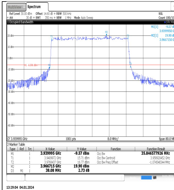
NTNV_N77-3700- 3980_PC2_30_40_H_TID2_Ant1#1
