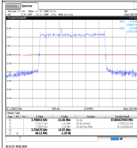
NTNV_N77-3700- 3980_PC2_30_60_L_TID3_Ant1#1
