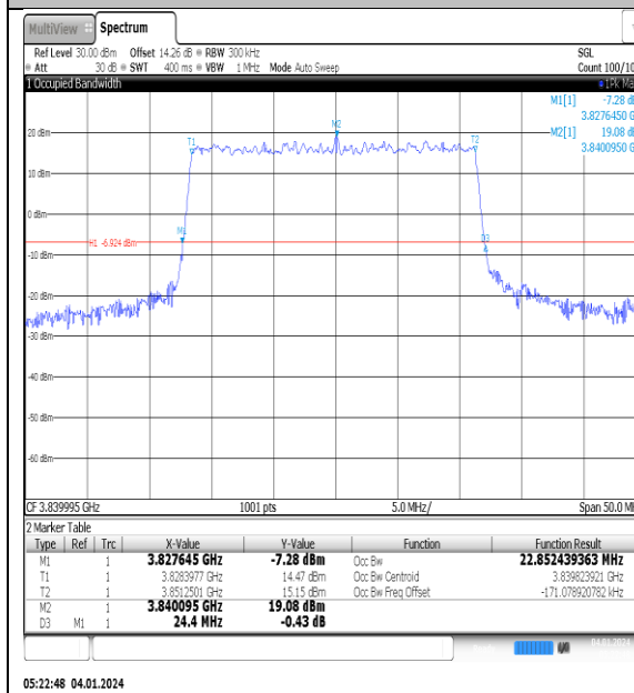
NTNV_N77-3700- 3980_PC2_30_25_M_TID2_Ant1#1
