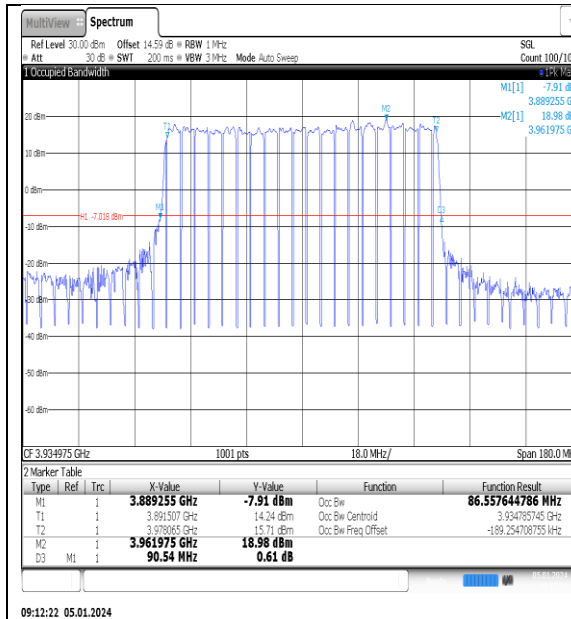
NTNV_N77-3700- 3980_PC2_30_90_H_TID1_Ant1#1
