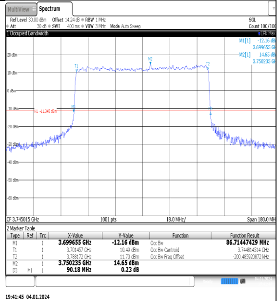
NTNV_N77-3700- 3980_PC2_30_90_L_TID4_Ant1#1
