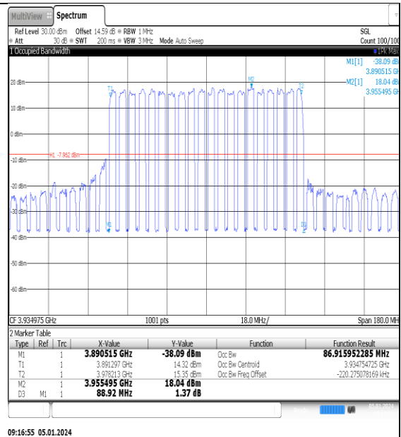
NTNV_N77-3700- 3980_PC2_30_90_H_TID2_Ant1#1
