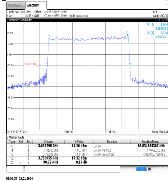
NTNV_N77-3700- 3980_PC2_30_90_L_TID3_Ant1#1
