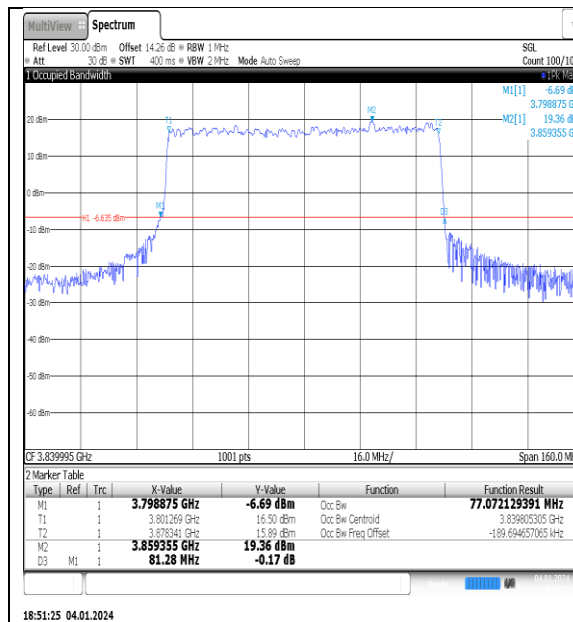
NTNV_N77-3700- 3980_PC2_30_80_M_TID1_Ant1#1
