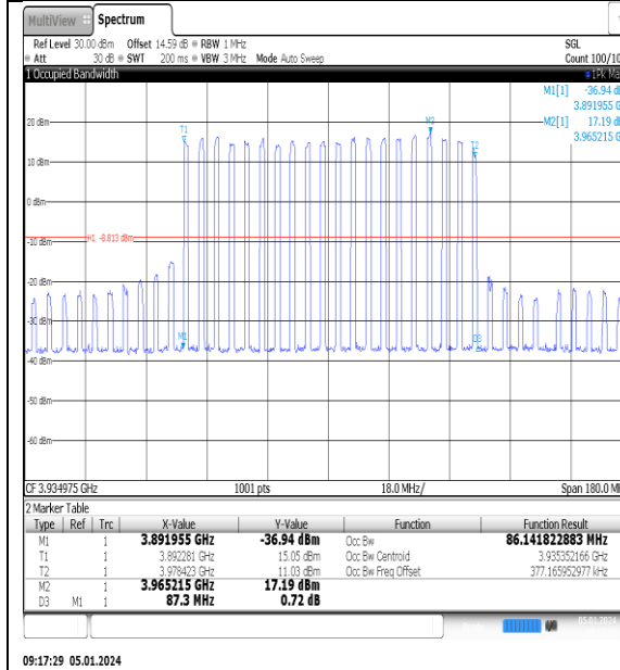
NTNV_N77-3700- 3980_PC2_30_90_H_TID3_Ant1#1
