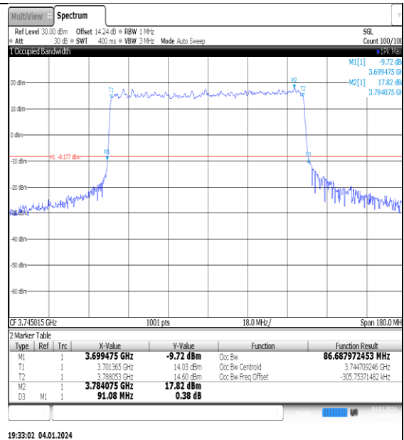
NTNV_N77-3700- 3980_PC2_30_90_L_TID2_Ant1#1
