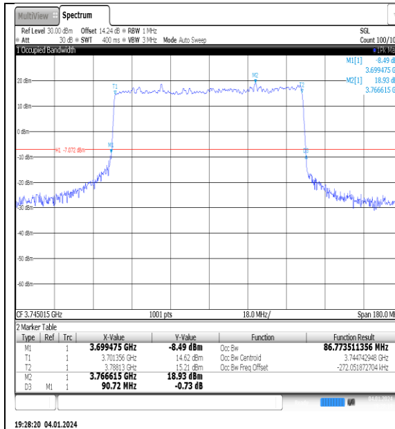
NTNV_N77-3700- 3980_PC2_30_90_L_TID1_Ant1#1
