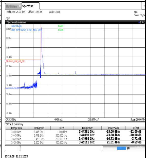
NTNV_N77-3450-3550_PC2_30_50_L_TID2_#1
