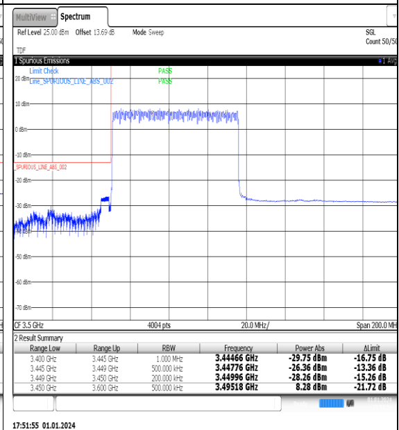
NTNV_N77-3450-3550_PC2_30_70_L_TID1_#1
