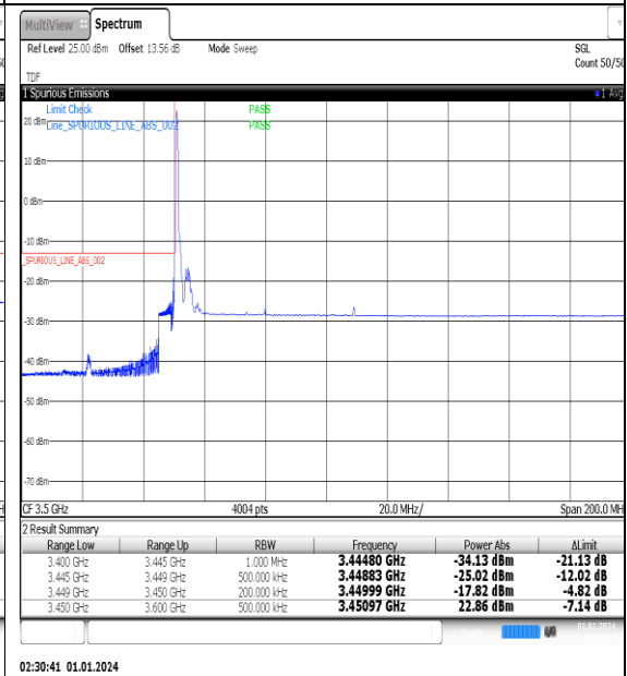
NTNV_N77-3450-3550_PC2_30_60_L_TID2_#1
