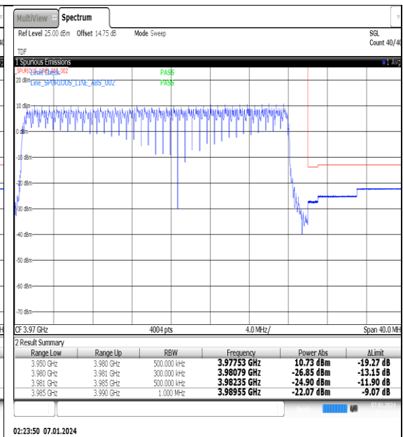
NTNV_N77-3700-3980_PC2_30_30_H_TID13_#1
