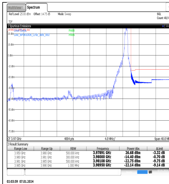
NTNV_N77-3700-3980_PC2_30_30_H_TID6_#1
