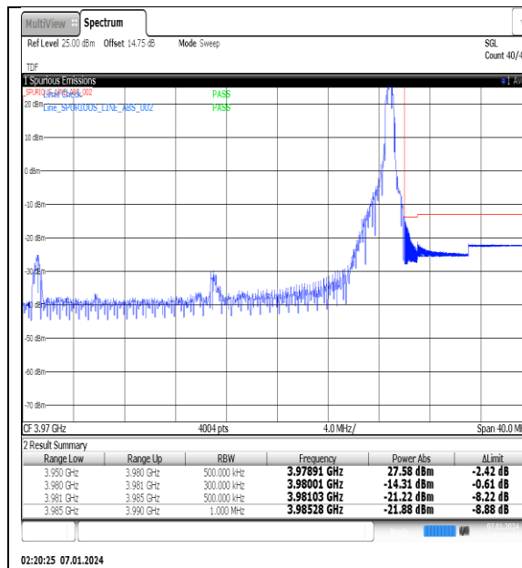
NTNV_N77-3700-3980_PC2_30_30_H_TID12_#1
