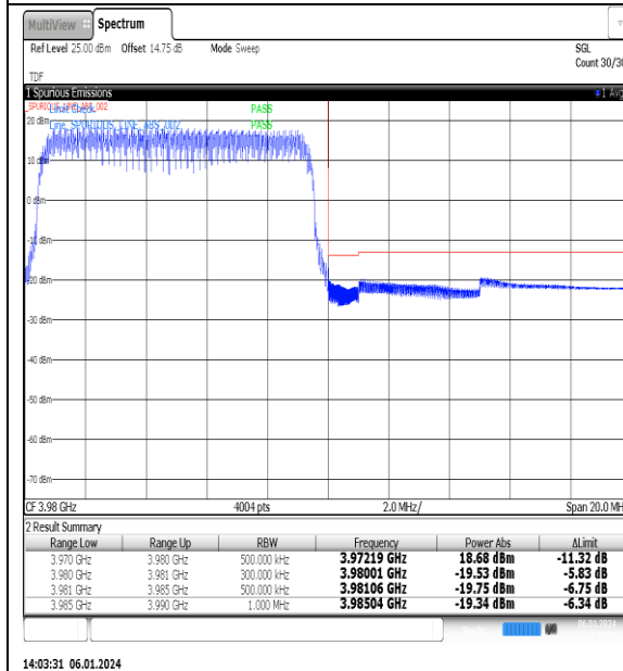
NTNV_N77-3700-3980_PC2_30_10_H_TID7_#1
