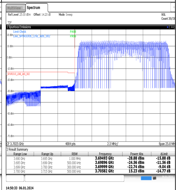
NTNV_N77-3700-3980_PC2_30_15_L_TID13_#1
