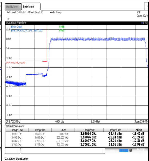
NTNV_N77-3700-3980_PC2_30_25_L_TID1_#1
