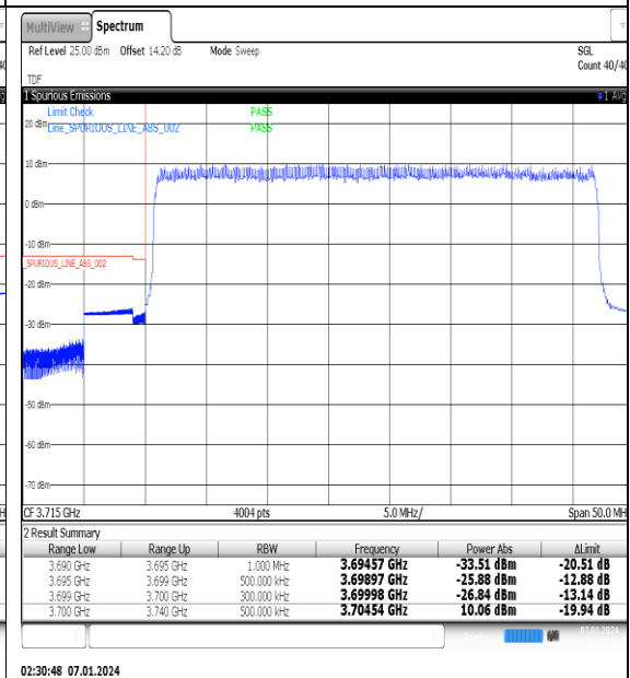
NTNV_N77-3700-3980_PC2_30_40_L_TID1_#1
