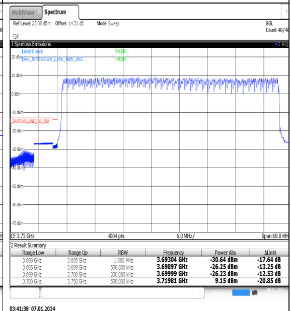
NTNV_N77-3700-3980_PC2_30_50_L_TID1_#1
