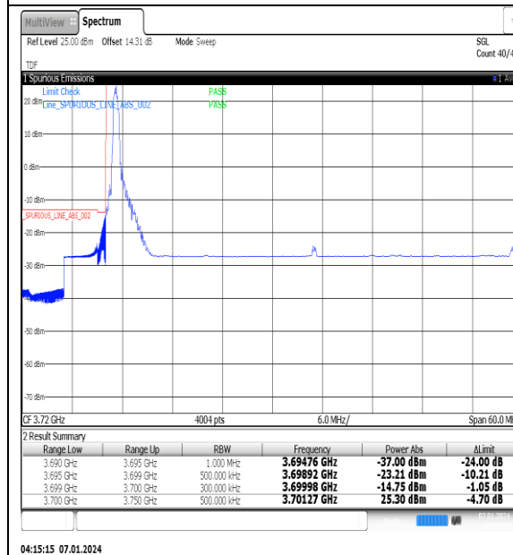
NTNV_N77-3700-3980_PC2_30_50_L_TID11_#1
