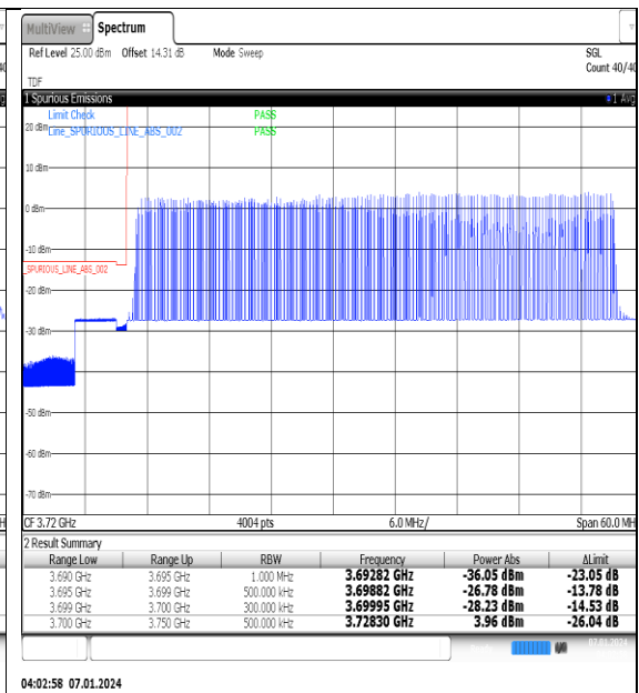
NTNV_N77-3700-3980_PC2_30_50_L_TID10_#1
