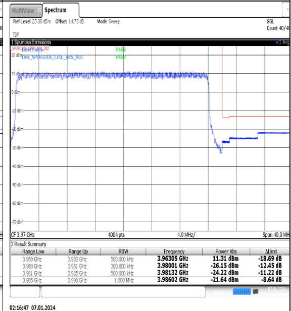
NTNV_N77-3700-3980_PC2_30_30_H_TID10_#1
