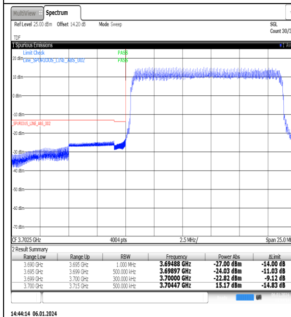
NTNV_N77-3700-3980_PC2_30_15_L_TID10_#1
