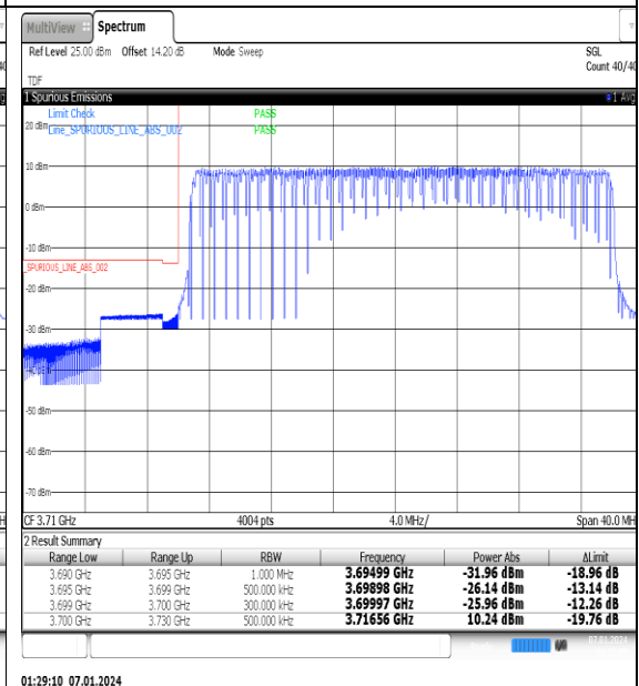
NTNV_N77-3700-3980_PC2_30_30_L_TID7_#1
