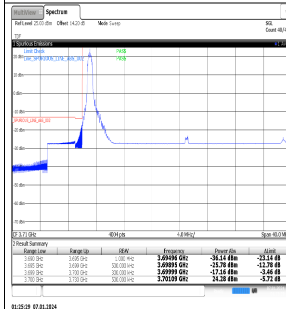
NTNV_N77-3700-3980_PC2_30_30_L_TID5_#1
