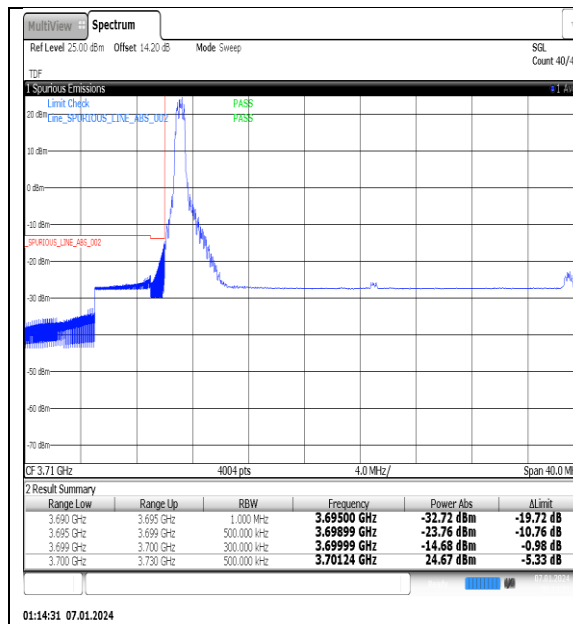
NTNV_N77-3700-3980_PC2_30_30_L_TID2_#1
