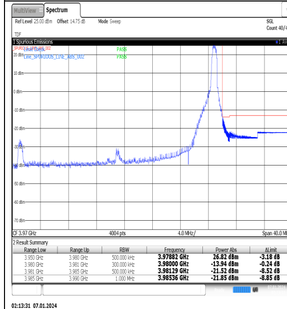
NTNV_N77-3700-3980_PC2_30_30_H_TID9_#1
