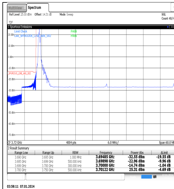
NTNV_N77-3700-3980_PC2_30_50_L_TID8_#1
