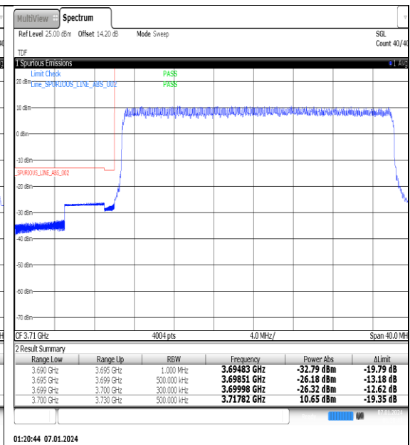
NTNV_N77-3700-3980_PC2_30_30_L_TID4_#1
