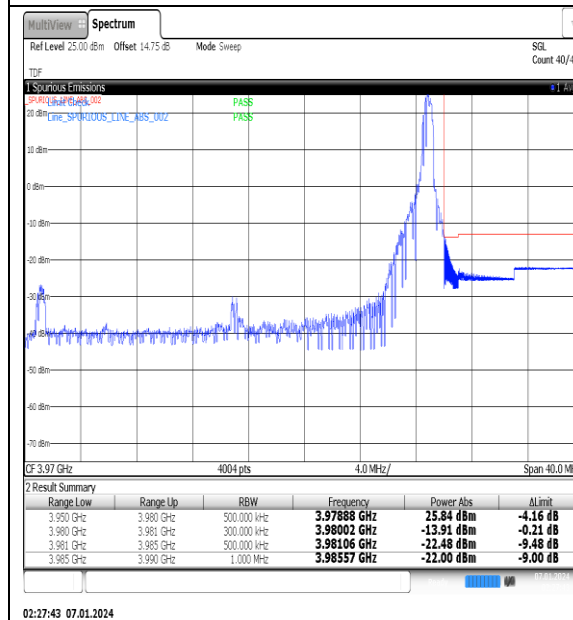
NTNV_N77-3700-3980_PC2_30_30_H_TID15_#1
