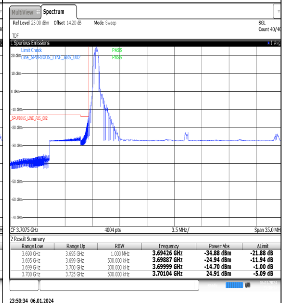
NTNV_N77-3700-3980_PC2_30_25_L_TID5_#1
