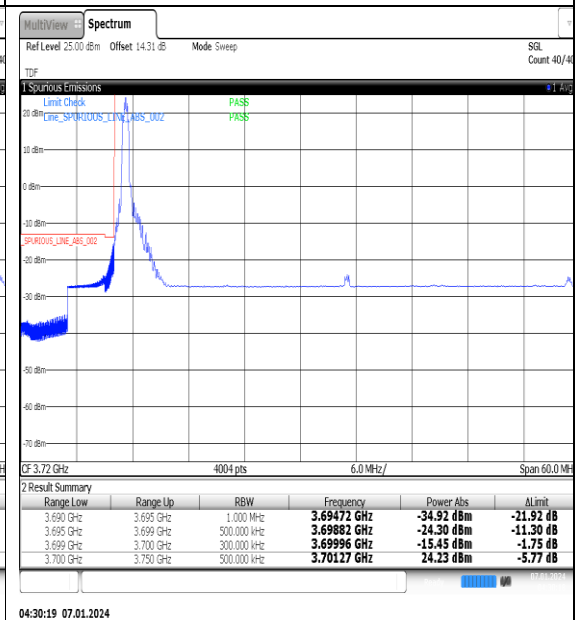
NTNV_N77-3700-3980_PC2_30_50_L_TID14_#1
