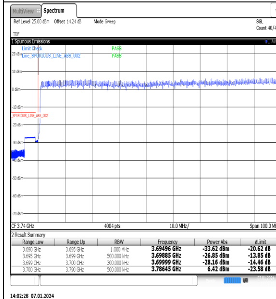
NTNV_N77-3700-3980_PC2_30_90_L_TID4_#1
