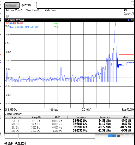
NTNV_N77-3700-3980_PC2_30_70_L_TID1_#1
