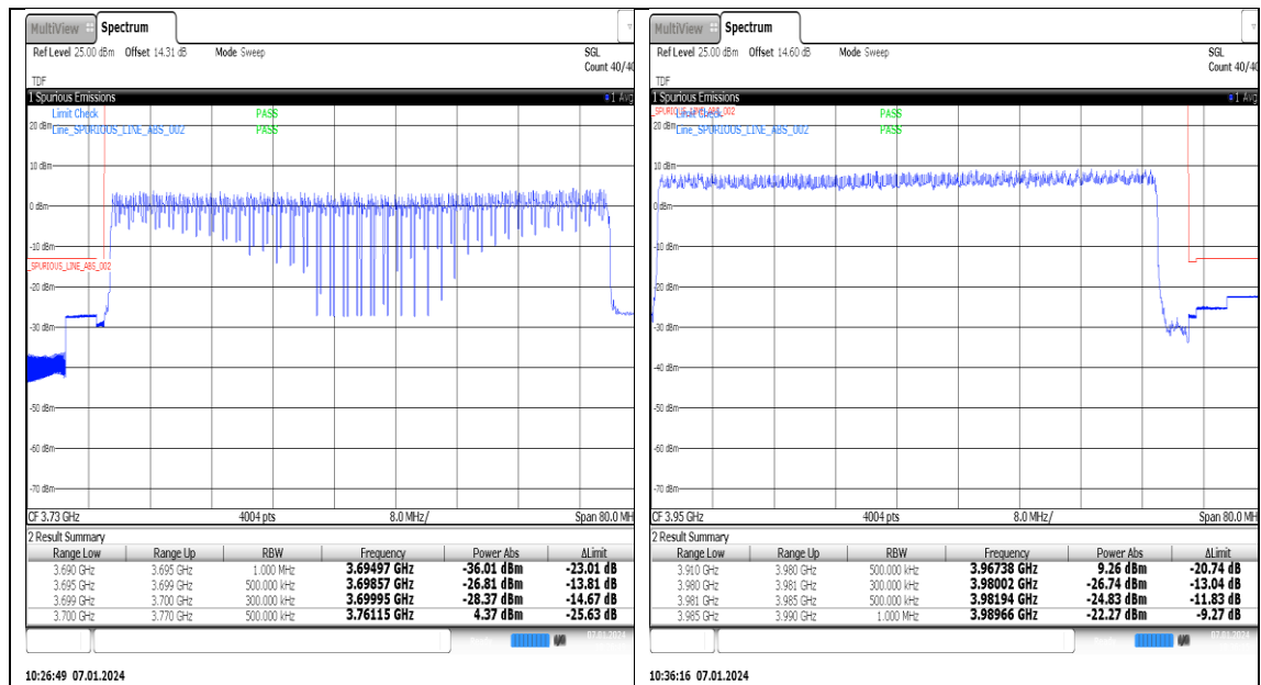
NTNV_N77-3700-3980_PC2_30_70_H_TID1_#1
