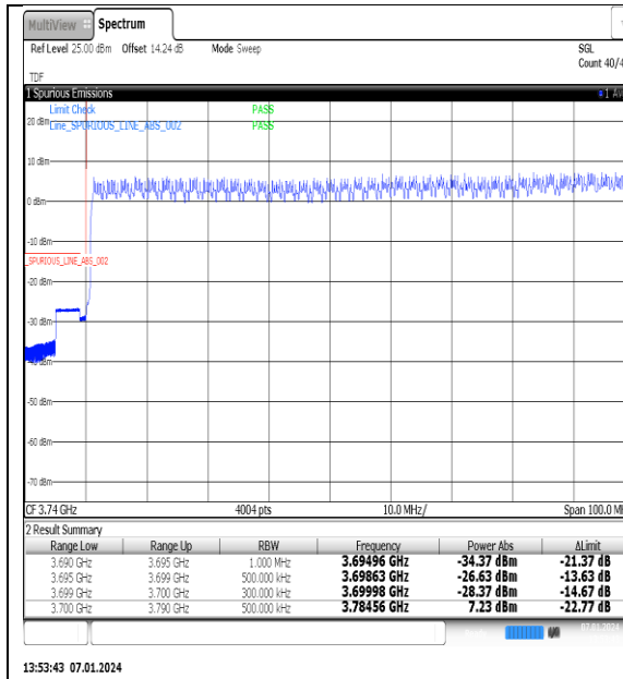
NTNV_N77-3700-3980_PC2_30_90_L_TID1_#1
