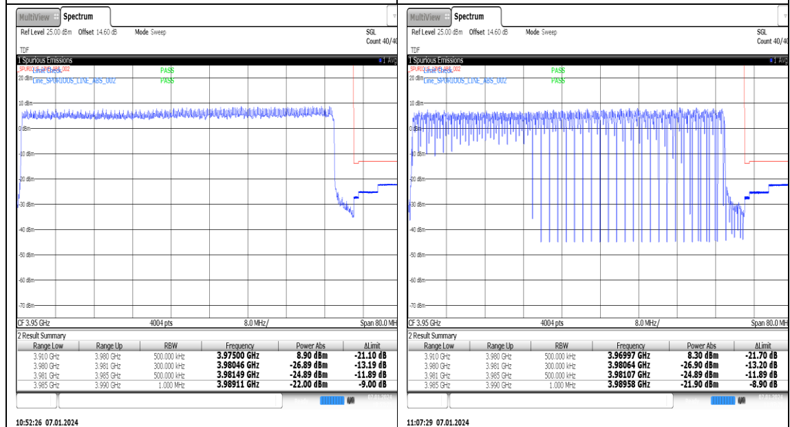
NTNV_N77-3700-3980_PC2_30_70_H_TID7_#1
