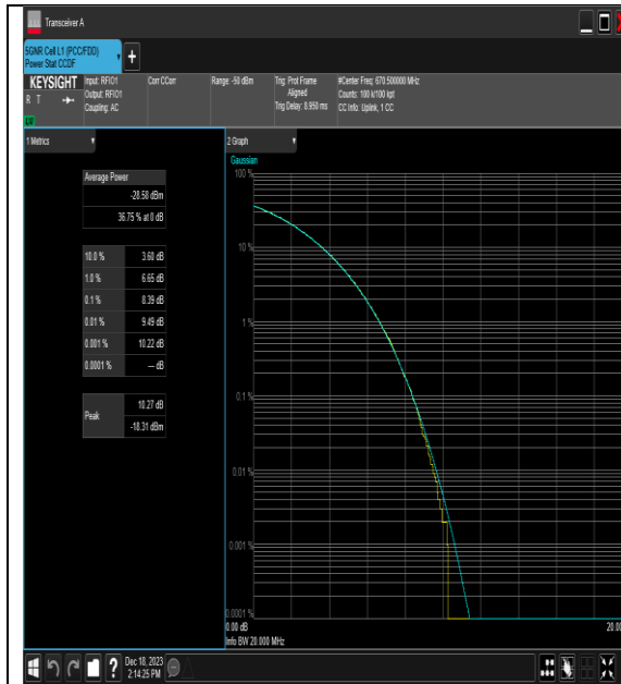
NTNV_N71_PC3_15_15_L_TID1_#1
