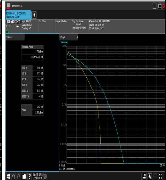
NTNV_N71_PC3_15_5_L_TID2_#1
