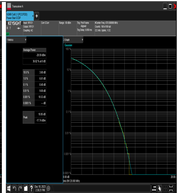
NTNV_N71_PC3_15_15_L_TID2_#1
