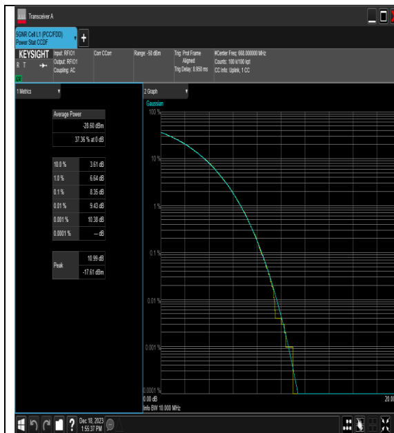
NTNV_N71_PC3_15_10_L_TID4_#1
