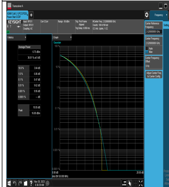
NTNV_N7_PC3_15_40_L_TID8_#1
