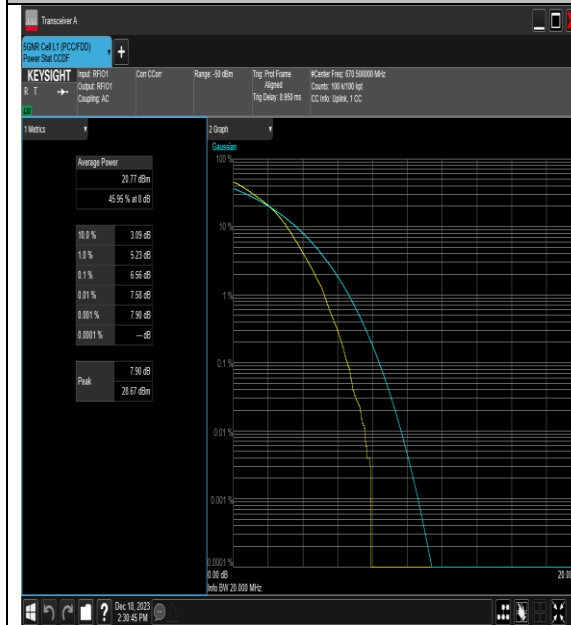
NTNV_N71_PC3_15_15_L_TID3_#1
