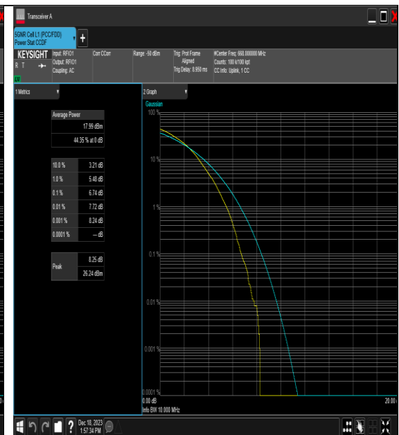
NTNV_N71_PC3_15_10_L_TID5_#1
