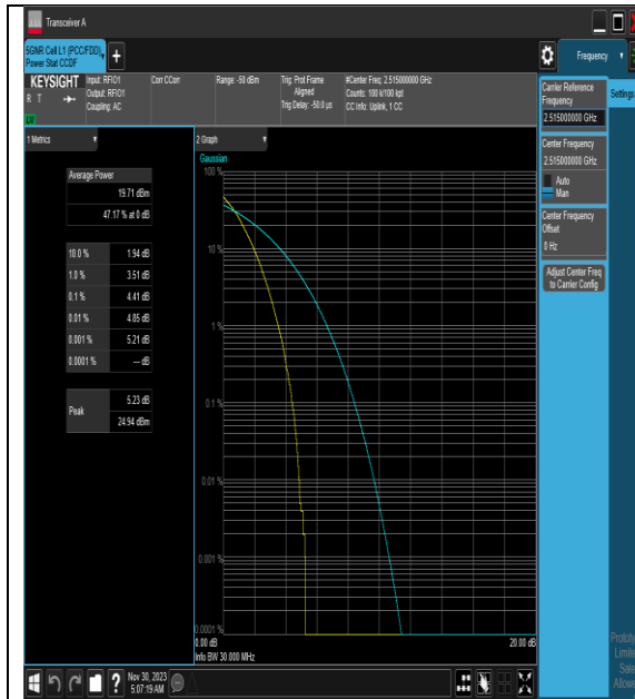
NTNV_N7_PC3_15_30_L_TID1_#1
