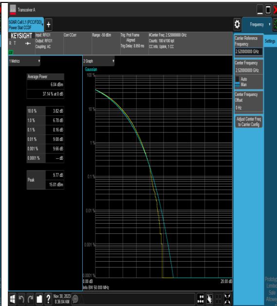
NTNV_N7_PC3_15_40_L_TID7_#1
