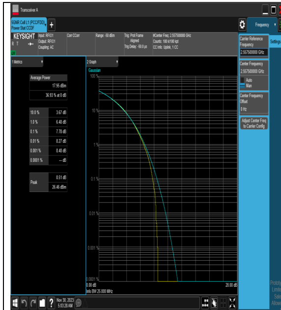
NTNV_N7_PC3_15_25_H_TID6_#1
