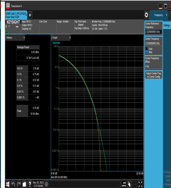
NTNV_N7_PC3_15_40_L_TID9_#1
