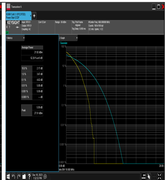
NTNV_N71_PC3_15_10_L_TID1_#1
