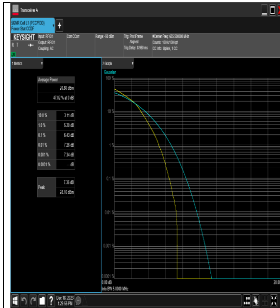
NTNV_N71_PC3_15_5_L_TID3_#1
