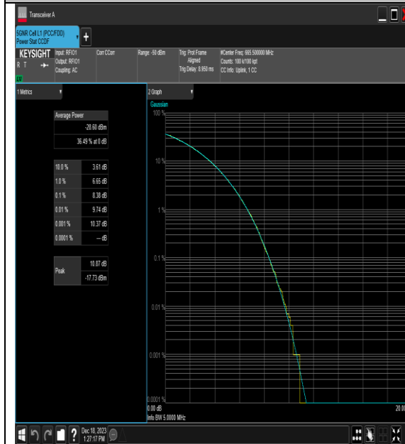
NTNV_N71_PC3_15_5_L_TID1_#1
