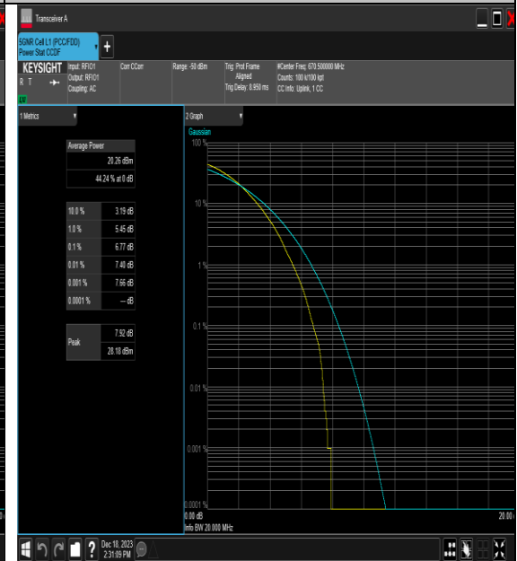
NTNV_N71_PC3_15_15_L_TID4_#1
