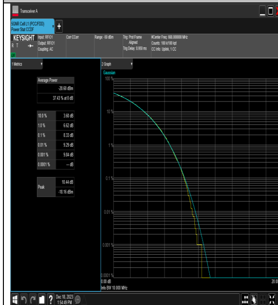
NTNV_N71_PC3_15_10_L_TID2_#1
