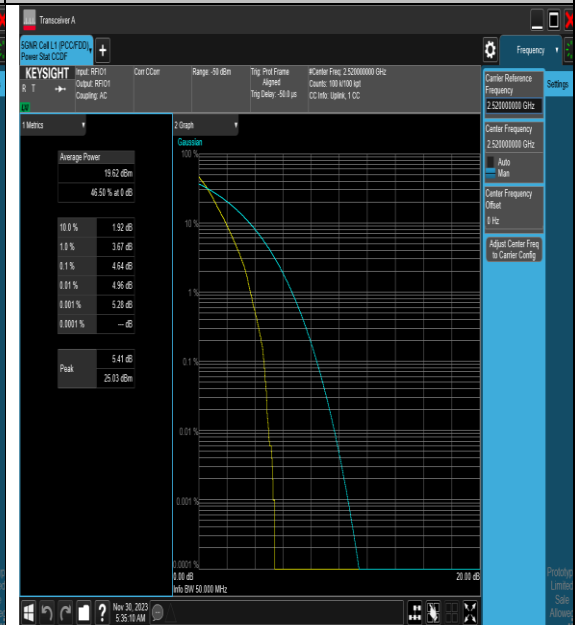
NTNV_N7_PC3_15_40_L_TID1_#1
