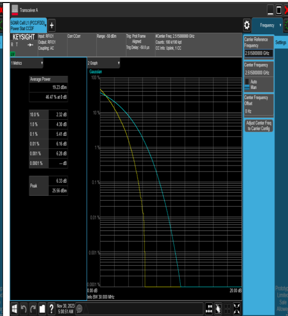
NTNV_N7_PC3_15_30_L_TID2_#1
