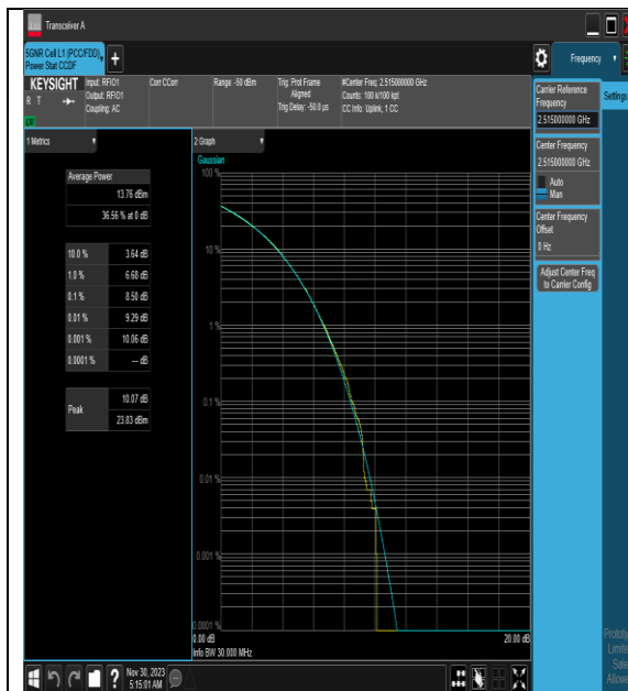
NTNV_N7_PC3_15_30_L_TID9_#1
