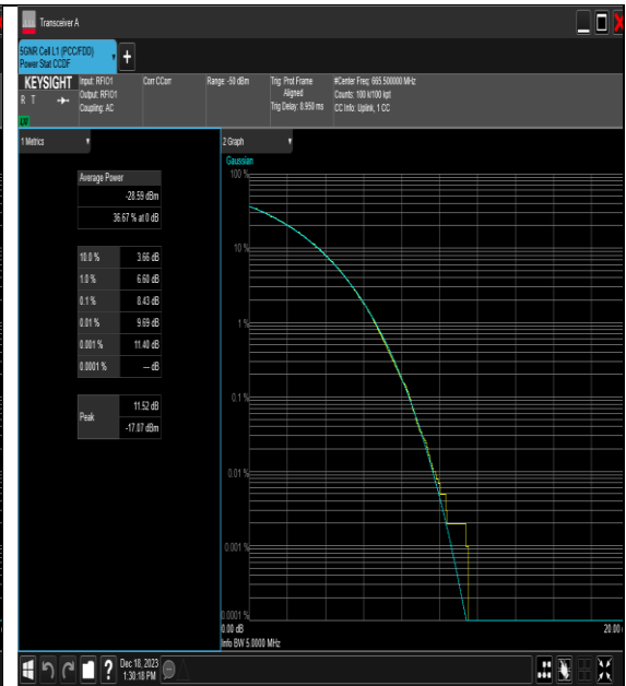
NTNV_N71_PC3_15_5_L_TID4_#1
