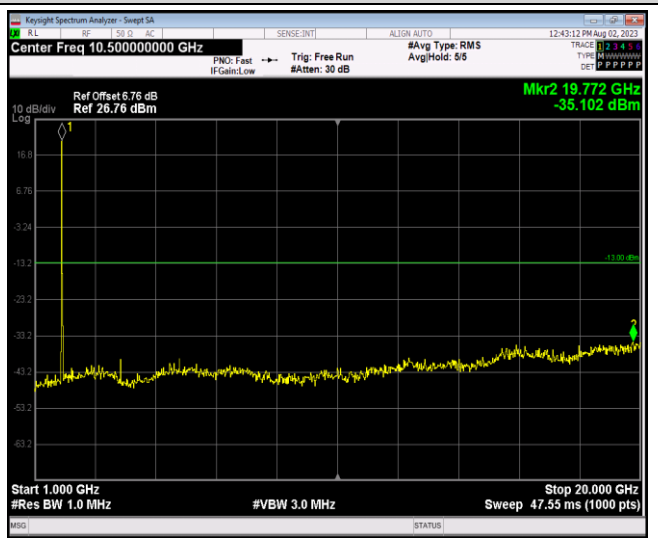
Band2-20MHz-QPSK-18700-1RB#0-Range2:1000~20000MHz
