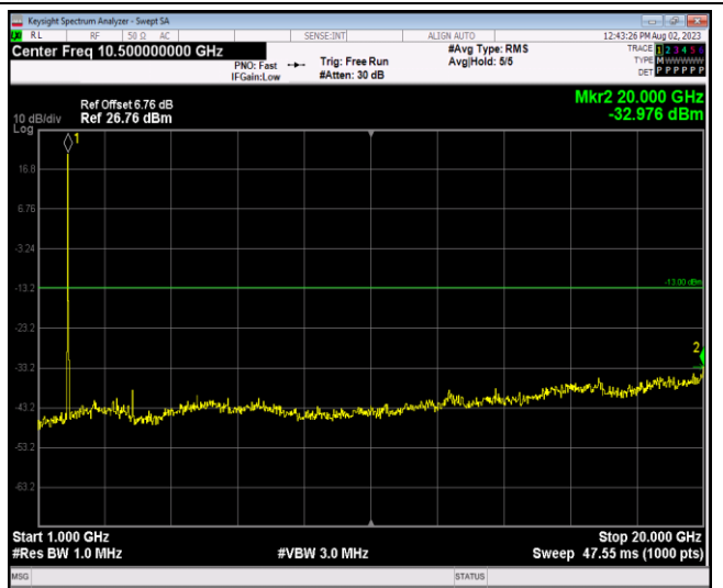
Band2-20MHz-16QAM-18900-1RB#0-Range2:1000~20000MHz
