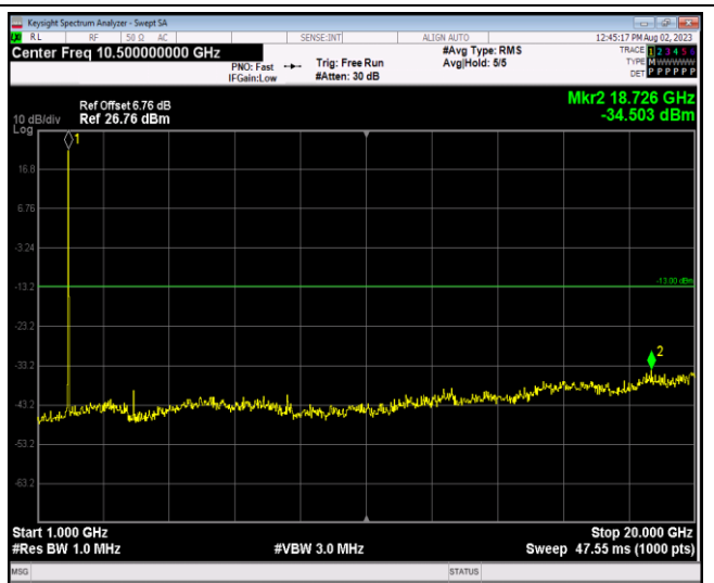
Band4-1.4MHz-QPSK-19957-1RB#0-Range2:1000~20000MHz
