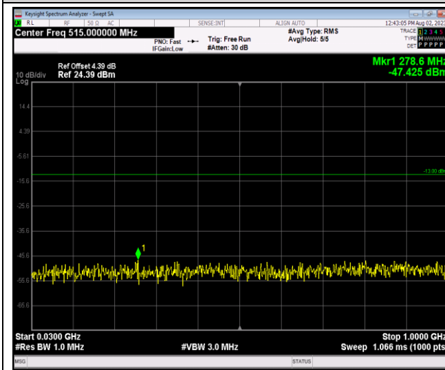
Band2-20MHz-QPSK-18700-1RB#0-Range1:30~1000MHz
