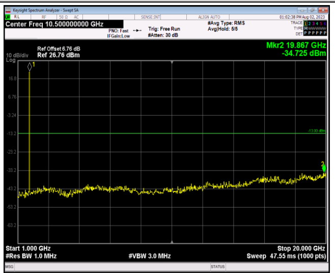
Band4-1.4MHz-QPSK-20175-1RB#0-Range2:1000~20000MHz
