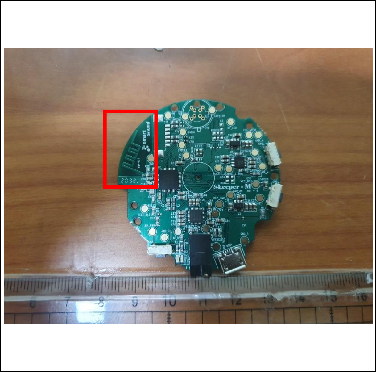
Antenna
