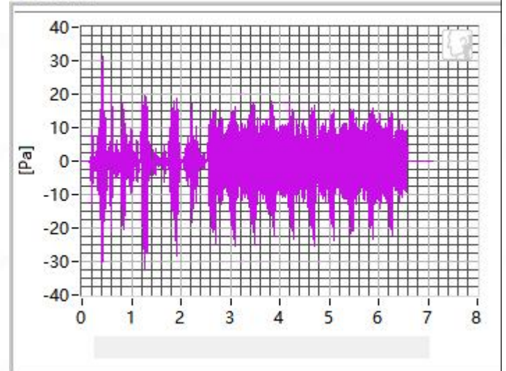
3150Hz
