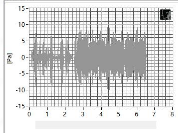
3150Hz
