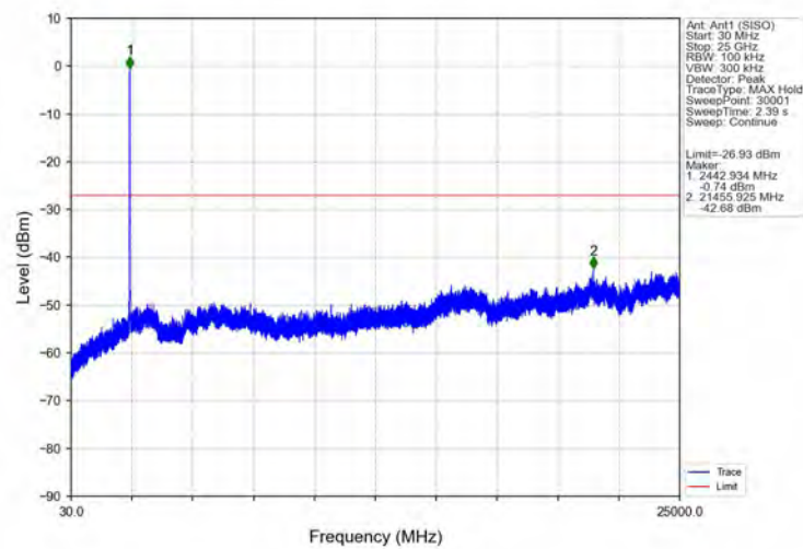
802.11g_MCH_2437MHz_Ant1 (SISO)_NTNV
