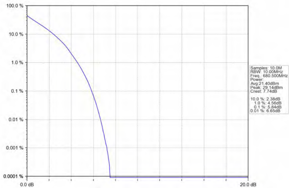
Band71_10MHz_QPSK_MCH_680.5MHz_RB_50_0_NTNV
