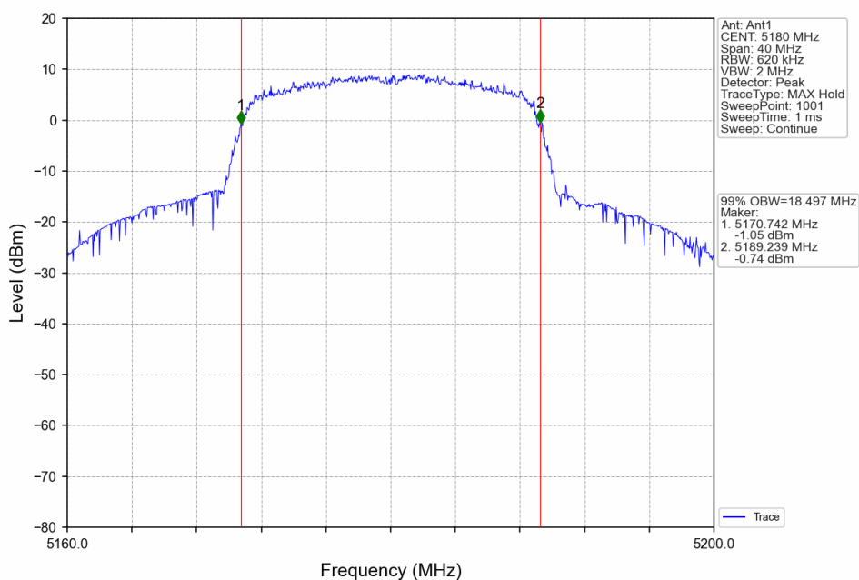
802.11n(HT20)_LCH_5180MHz_Ant1_NTNV
