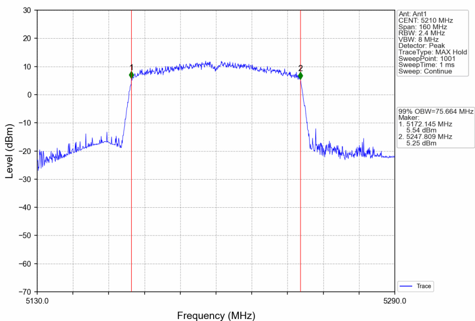
802.11ac(VHT80)_MCH_5210MHz_Ant1_NTNV
