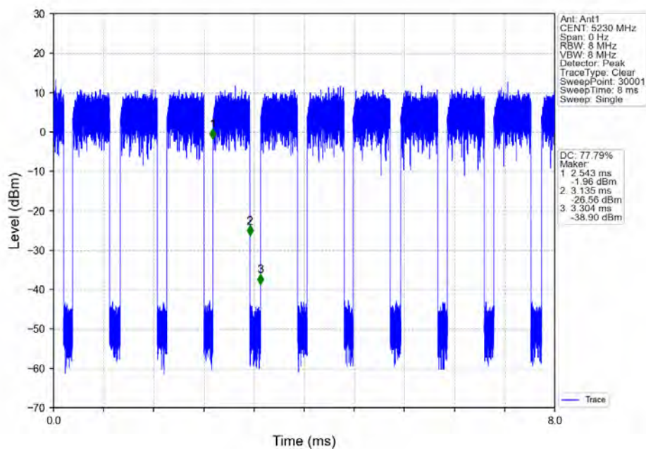
802.11ac(VHT40)_HCH_5230MHz_Ant1_NTNV
