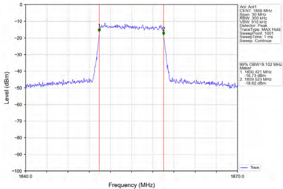
Band2_10MHz_16QAM_LCH_1855MHz_RB_50_0_NTNV
