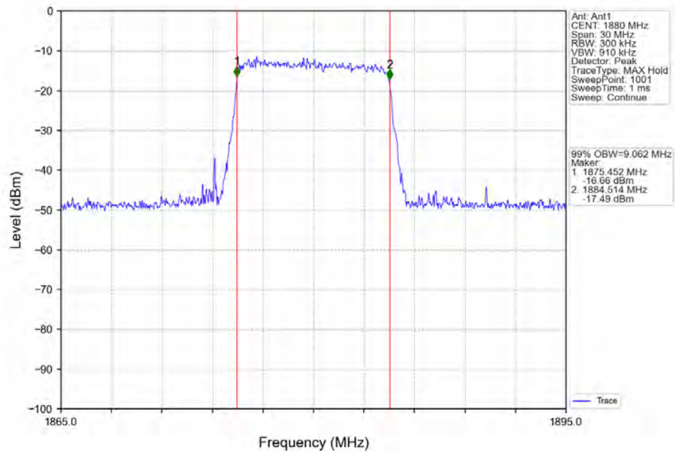
Band2_10MHz_QPSK_MCH_1880MHz_RB_50_0_NTNV
