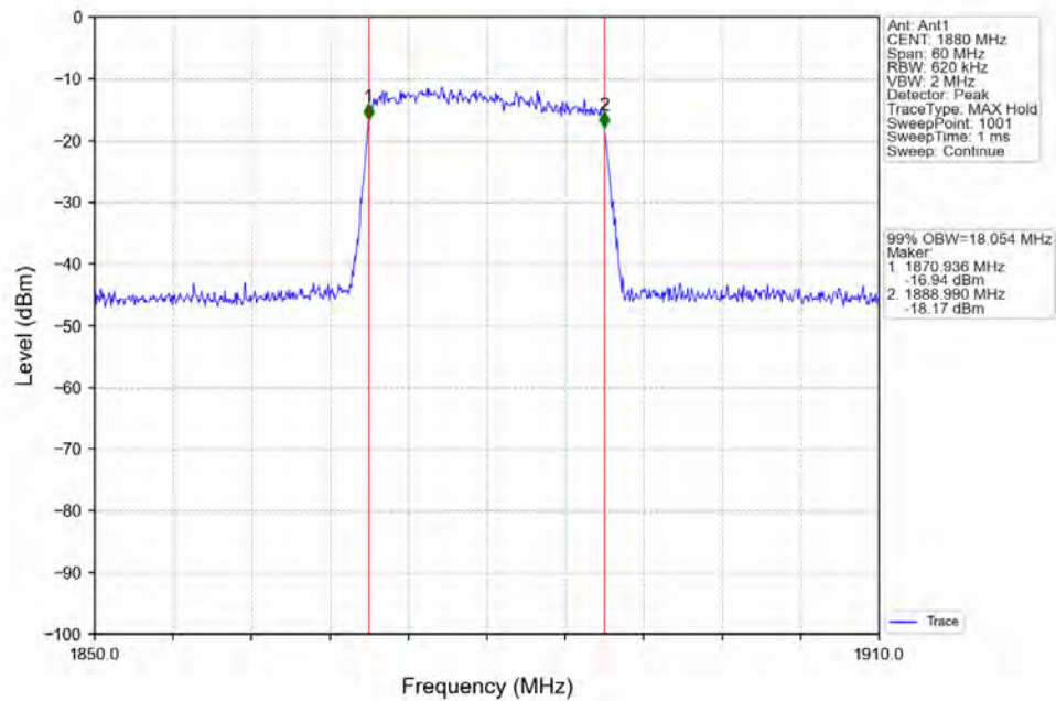
Band2_20MHz_QPSK_MCH_1880MHz_RB_100_0_NTNV
