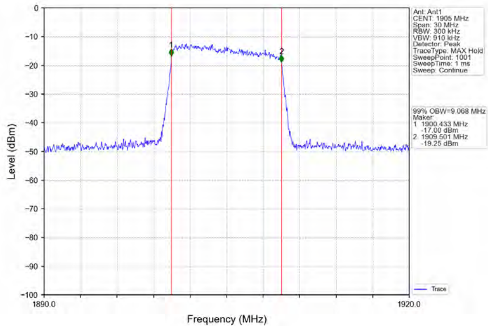
Band2_10MHz_16QAM_HCH_1905MHz_RB_50_0_NTNV
