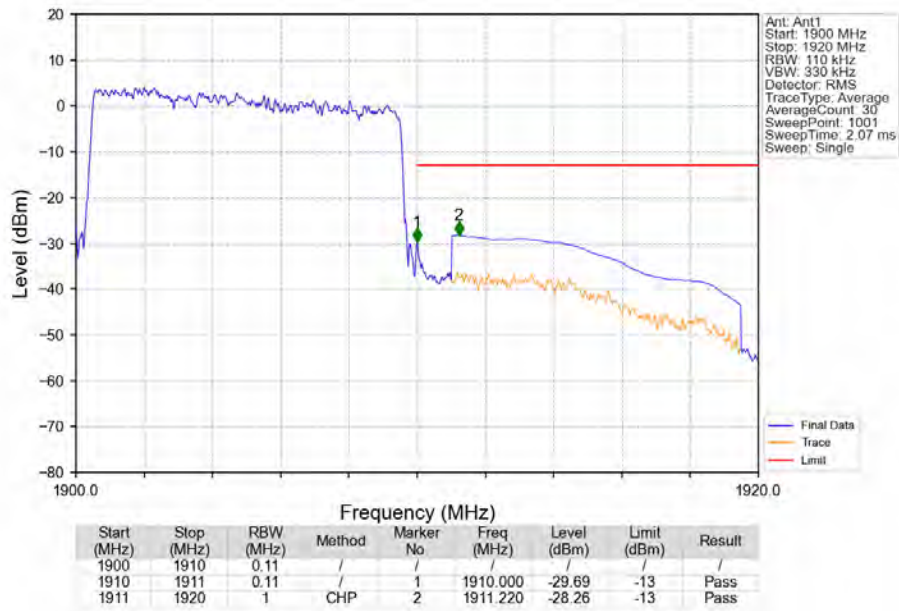
Band2_10MHz_QPSK_HCH_1905MHz_RB_50_0_NTNV
