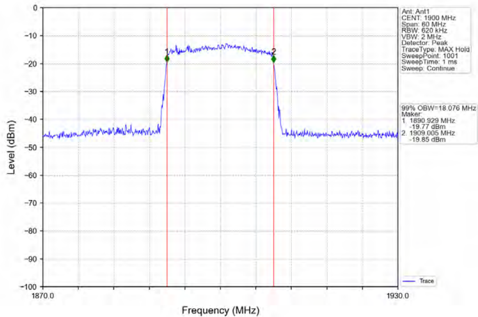
Band2_20MHz_16QAM_HCH_1900MHz_RB_100_0_NTNV
