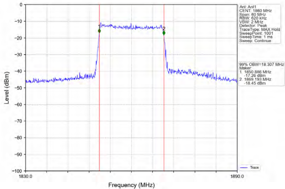
Band2_20MHz_16QAM_LCH_1860MHz_RB_100_0_NTNV
