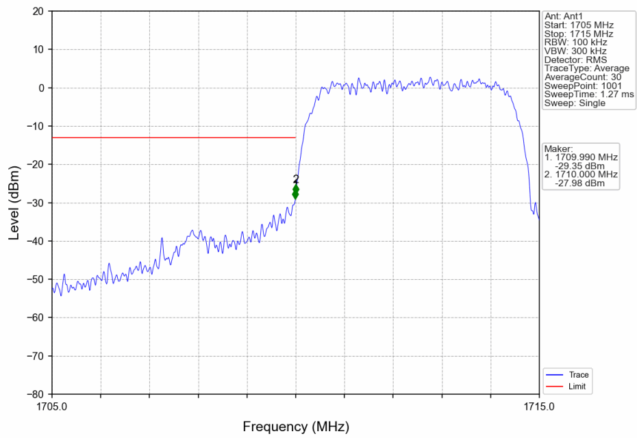
Band4_HSUPA_LCH_1712.4MHz_Subtest 1_NTNV
