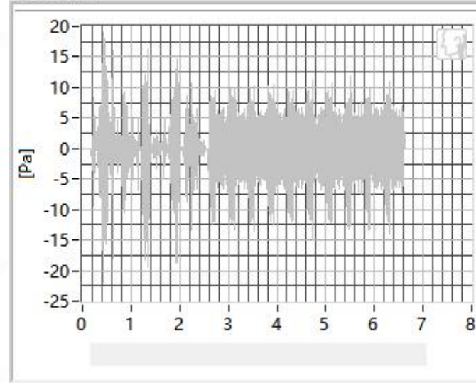
1250Hz
