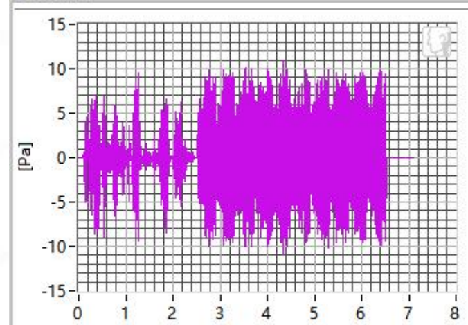
3150Hz
