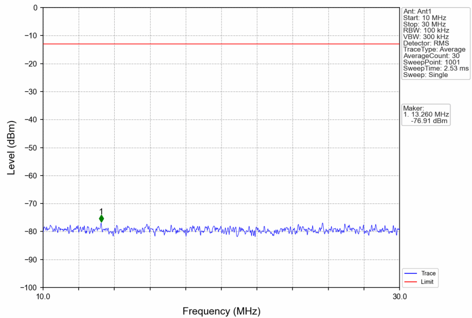
Band26a_10MHz_QPSK_MCH_819MHz_RB_1_0_NTNV
