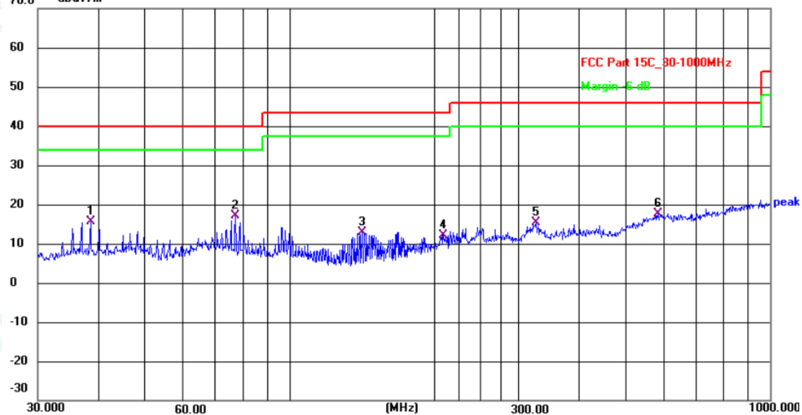
Horizontal 70.0 dBuV/m
