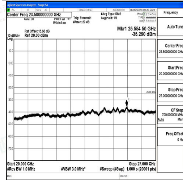
Band41_15MHz_QPSK_39725_1RB#0_20000~27000_2 0000~27000
