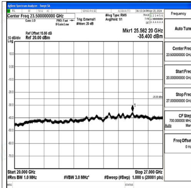
Band41_15MHz_QPSK_41515_1RB#0_20000~27000_2 0000~27000
