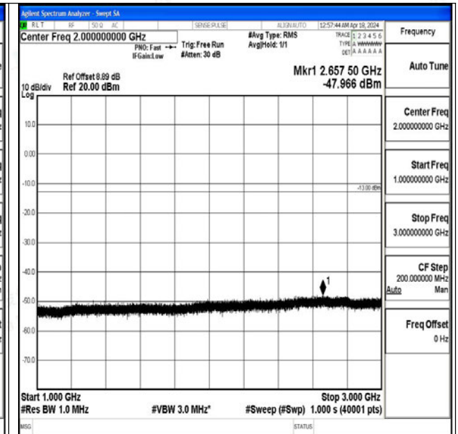
Band71_10MHz_QPSK_133172_1RB#0_1000~3000_1000~3000
