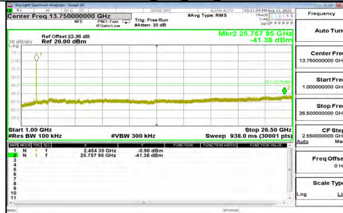
11N20SISO Ant1 2462 1000~26500
