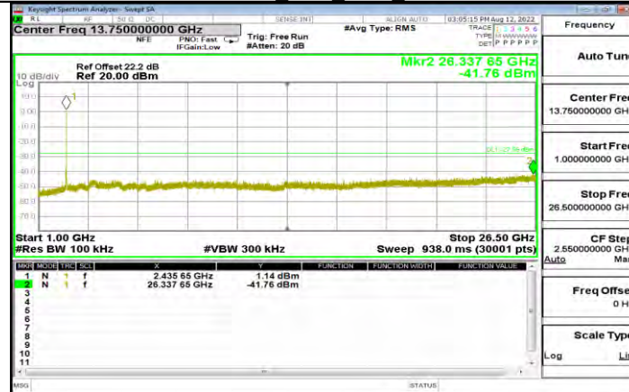
11N20SISO Ant1 2437 1000~26500
