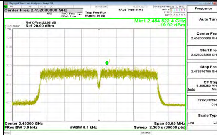
11N40SISO Ant1 2452
