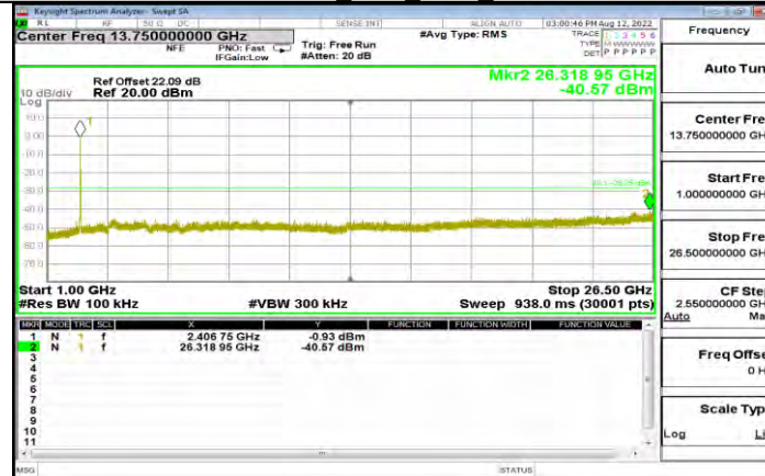
11N20SISO Ant1 2412 1000~26500
