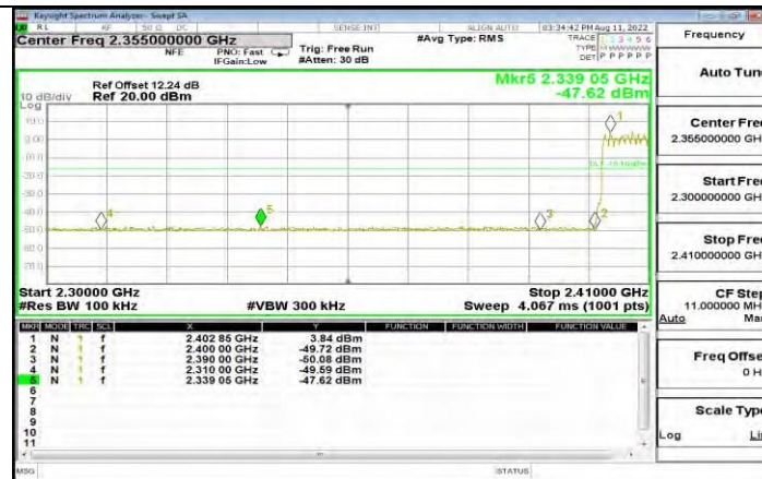
3DH5_Ant1_Low_Hop_2402
