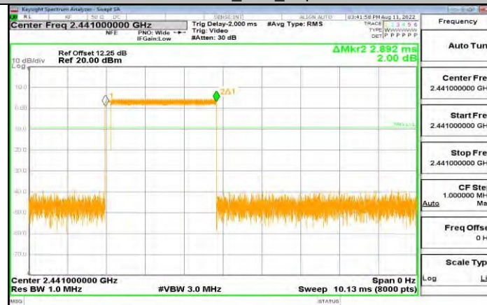
3DH5_Ant1_Hop
