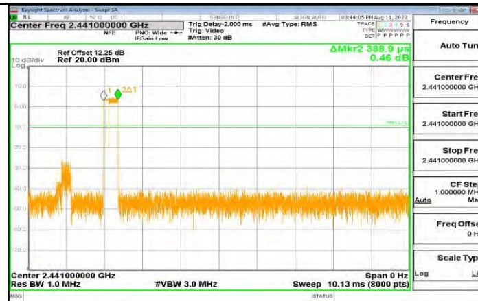
3DH1_Ant1_Hop
