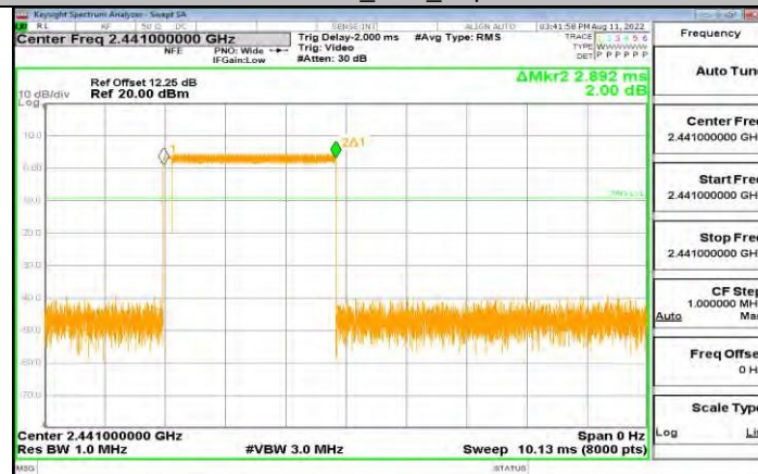
3DH5_Ant1_Hop
