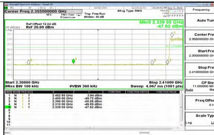
3DH5_Ant1_Low_Hop_2402
