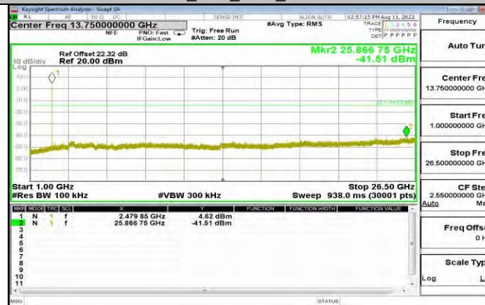
DH5_Ant1_2480_1000-26500
