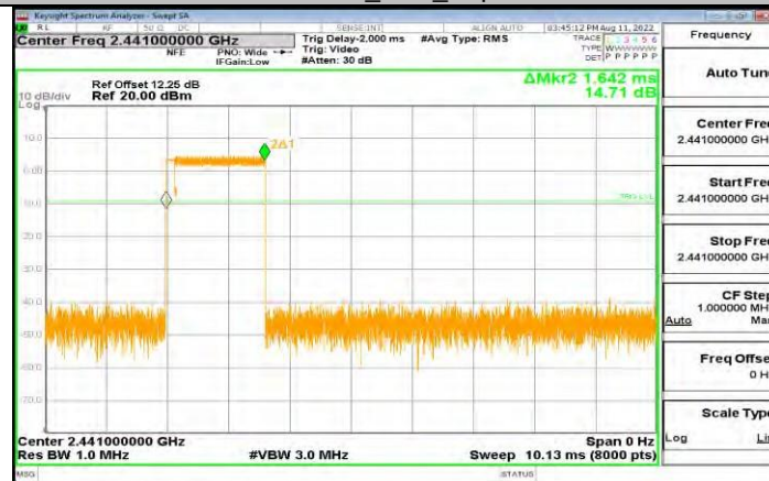
3DH3_Ant1_Hop
