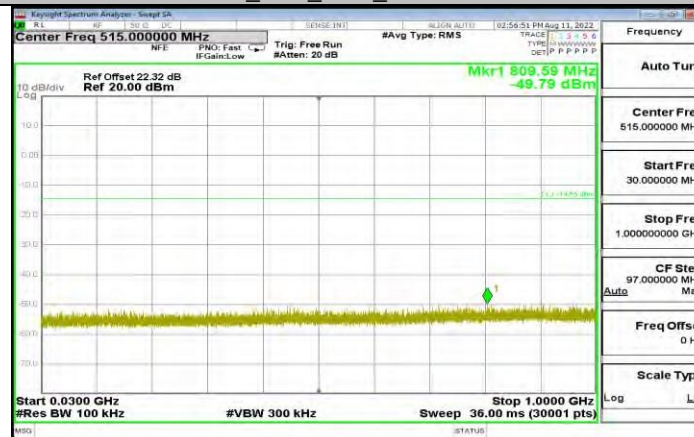
DH5_Ant1_2480_30-1000
