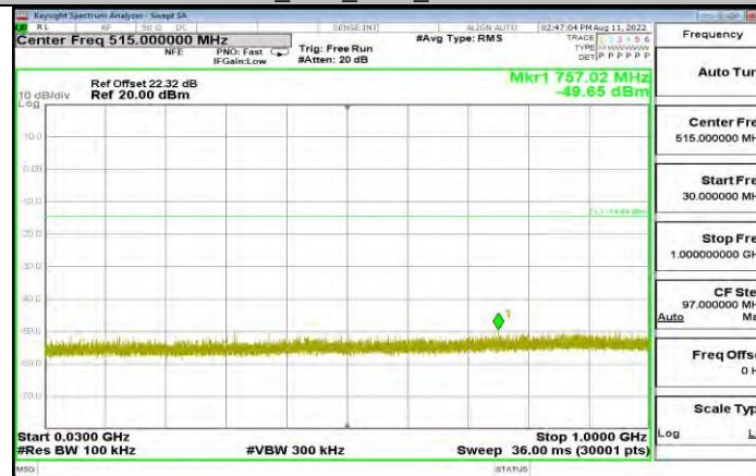
3DH5_Ant1_2480_30-1000
