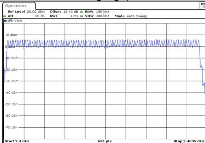
2DH1_Ant1_Hop
