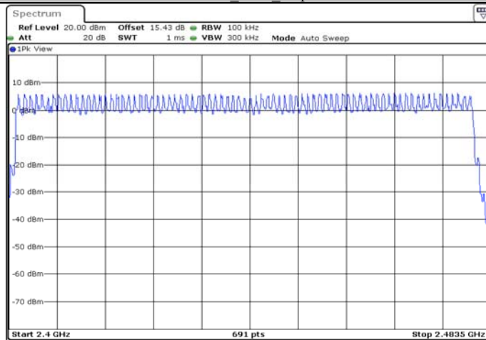
3DH1_Ant1_Hop
