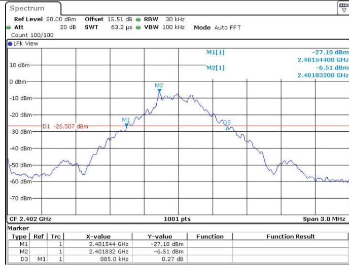
DH1_Ant1_2402
