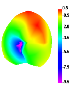
2400.000MHz E1
