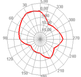
2500.000MHz
