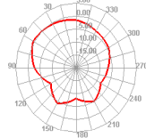
2450.000MHz H
