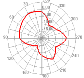
2450.000MHz
