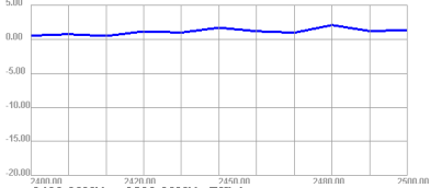
2400.00MHz - 2500.00MHz Efficiency
