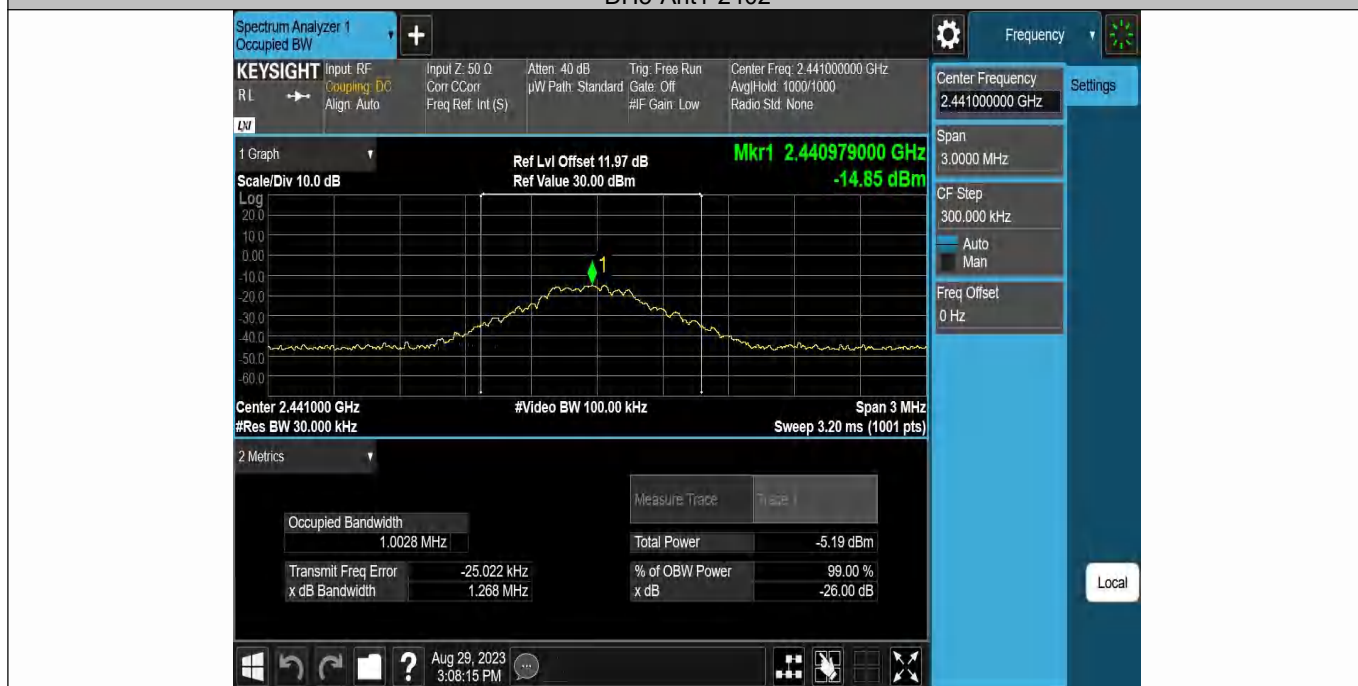
DH5-Ant1-2441
