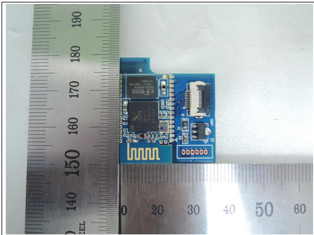
&lt;BT ANT&gt;
