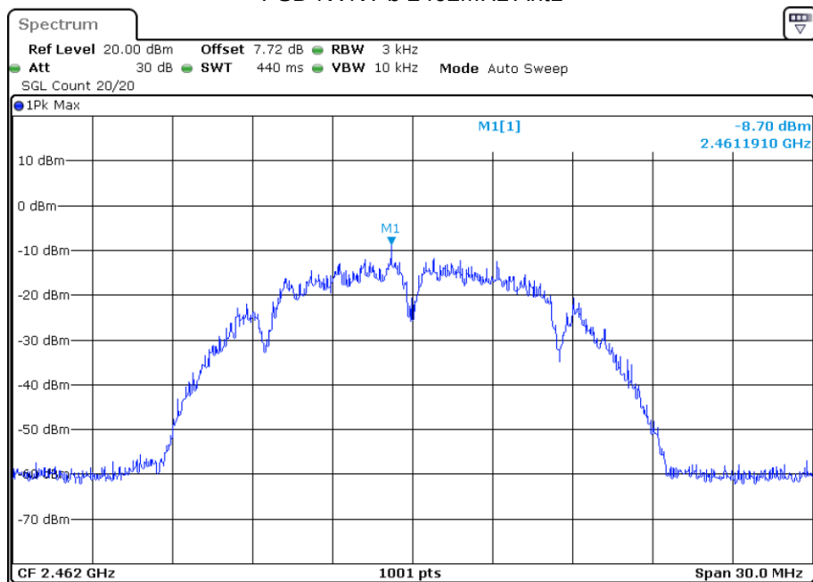
PSD NVNT b 2462MHz Ant1
