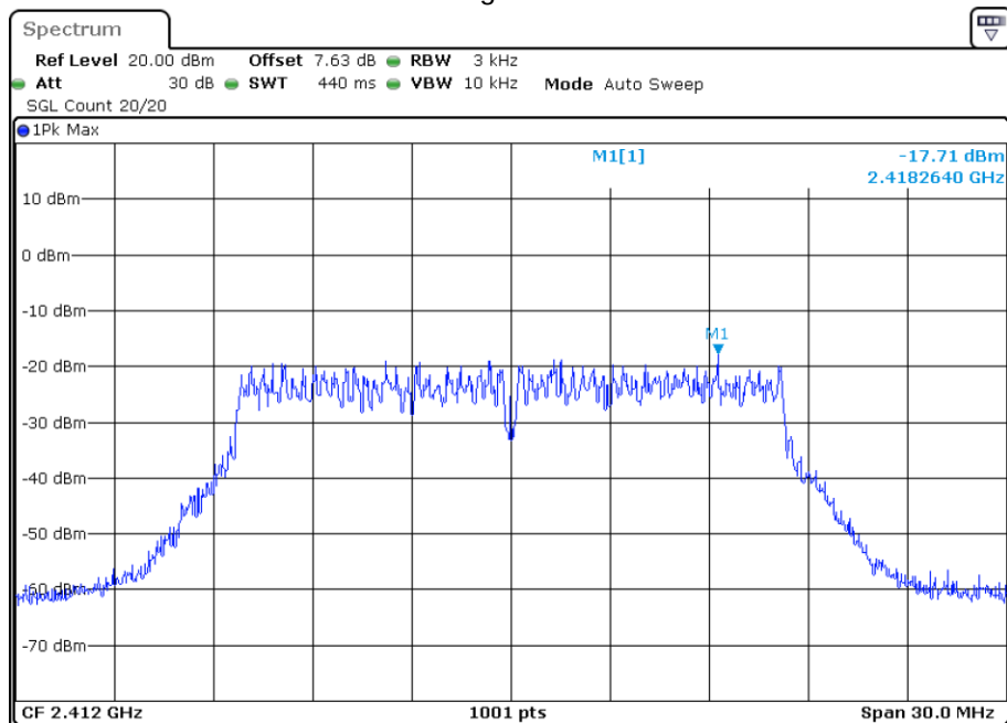
PSD NVNT g 2412MHz Ant1
