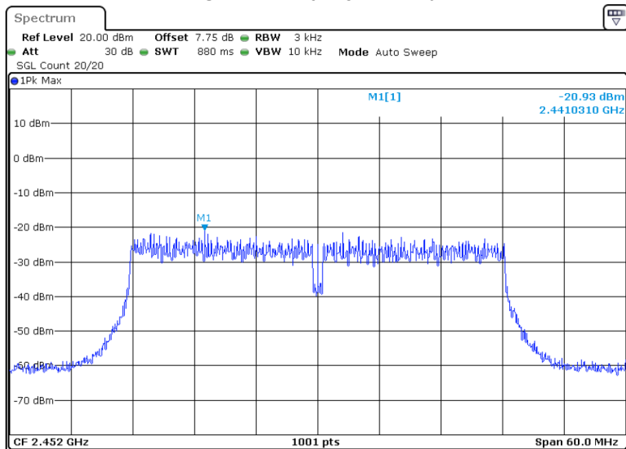
PSD NVNT n40 2452MHz Ant1
