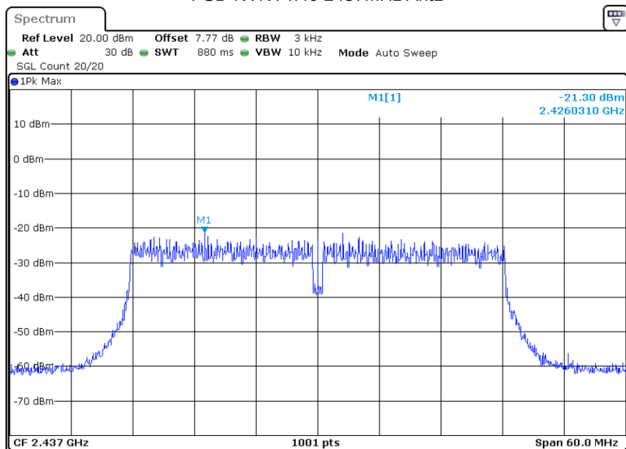
PSD NVNT n40 2437MHz Ant1
