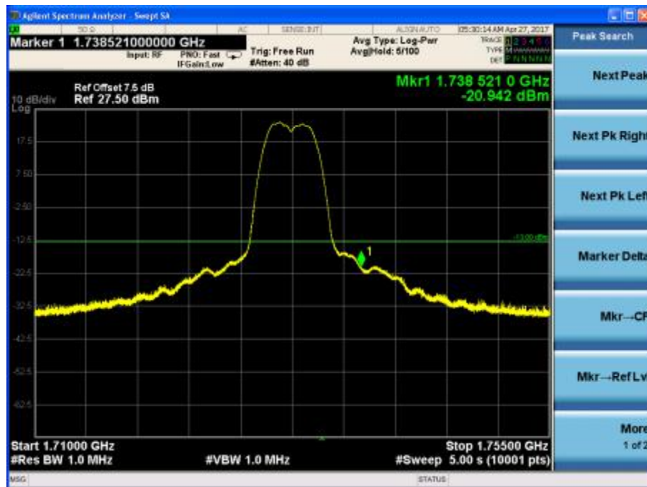
Channel 1412, 1710MHz~1755MHz
