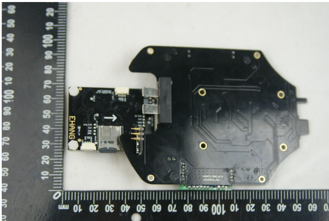
EUT PHOTO 20
