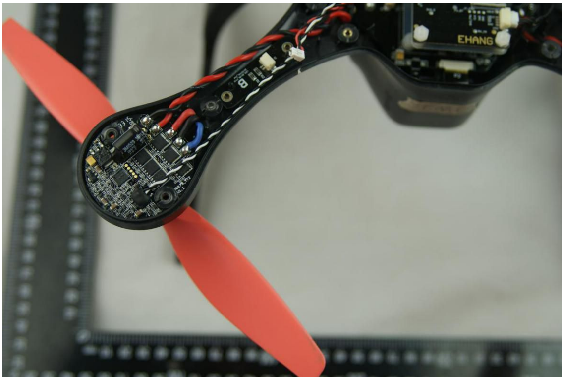
EUT PHOTO 14
