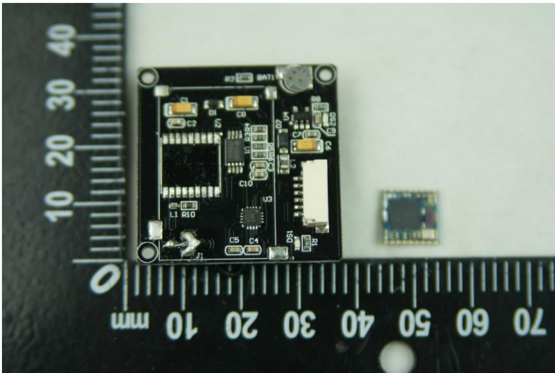
EUT PHOTO 10
