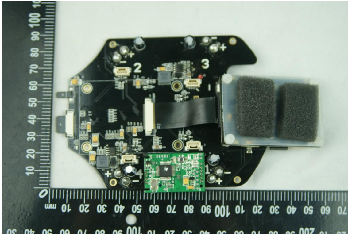
EUT PHOTO 19
