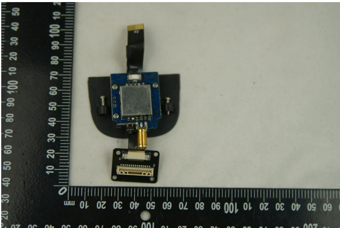
EUT PHOTO 32
