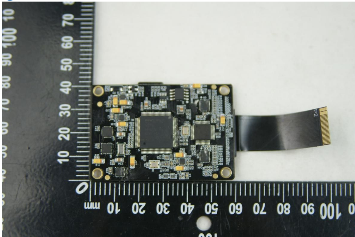
EUT PHOTO 45
