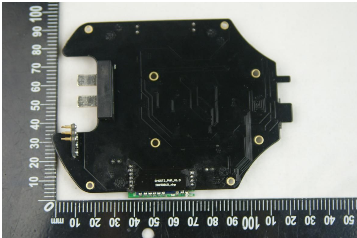
EUT PHOTO 22
