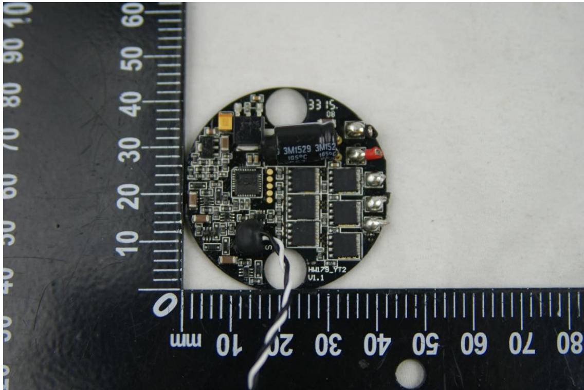
EUT PHOTO 17
