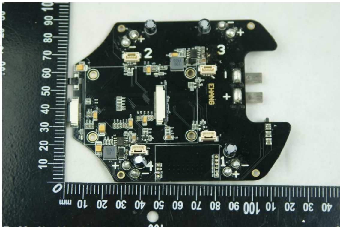
EUT PHOTO 24
