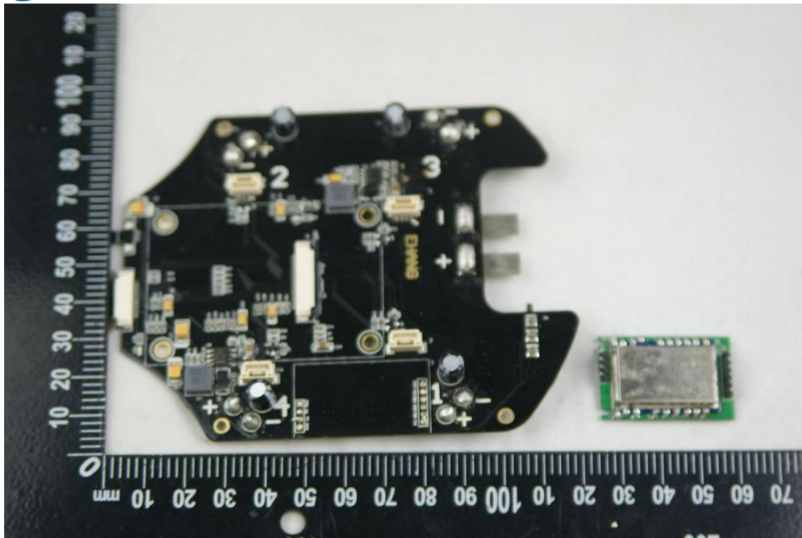
EUT PHOTO 23
