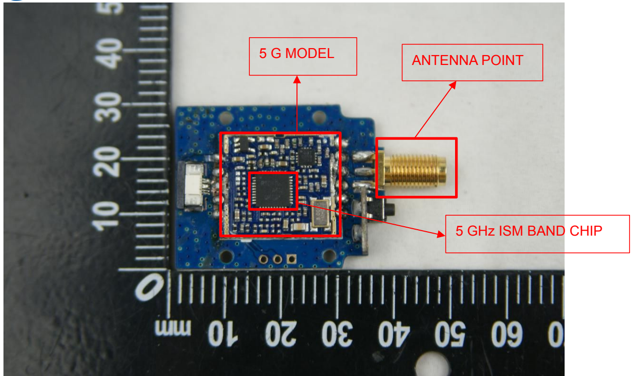
EUT PHOTO 39(5G model)
