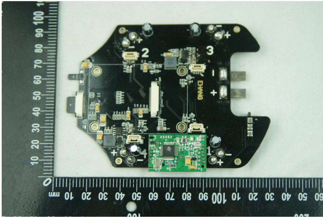
EUT PHOTO 21
