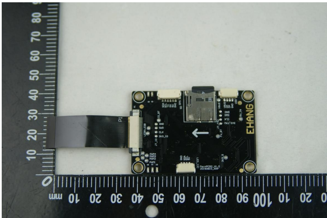
EUT PHOTO 46
