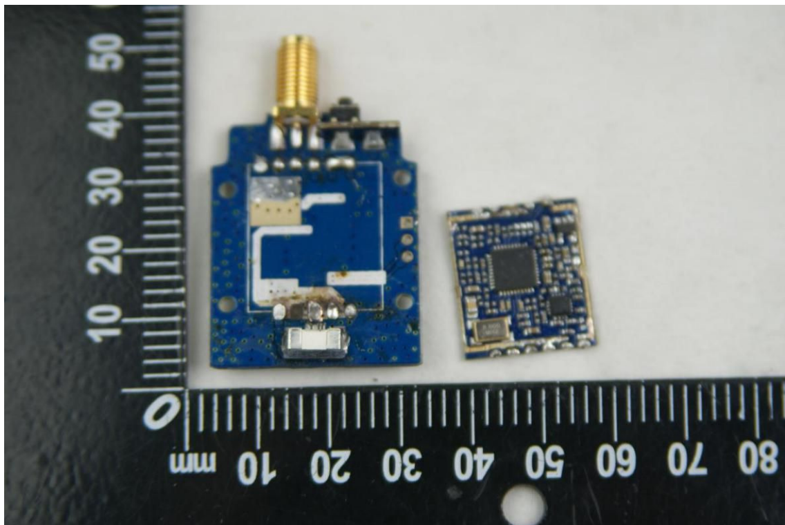
EUT PHOTO 40
