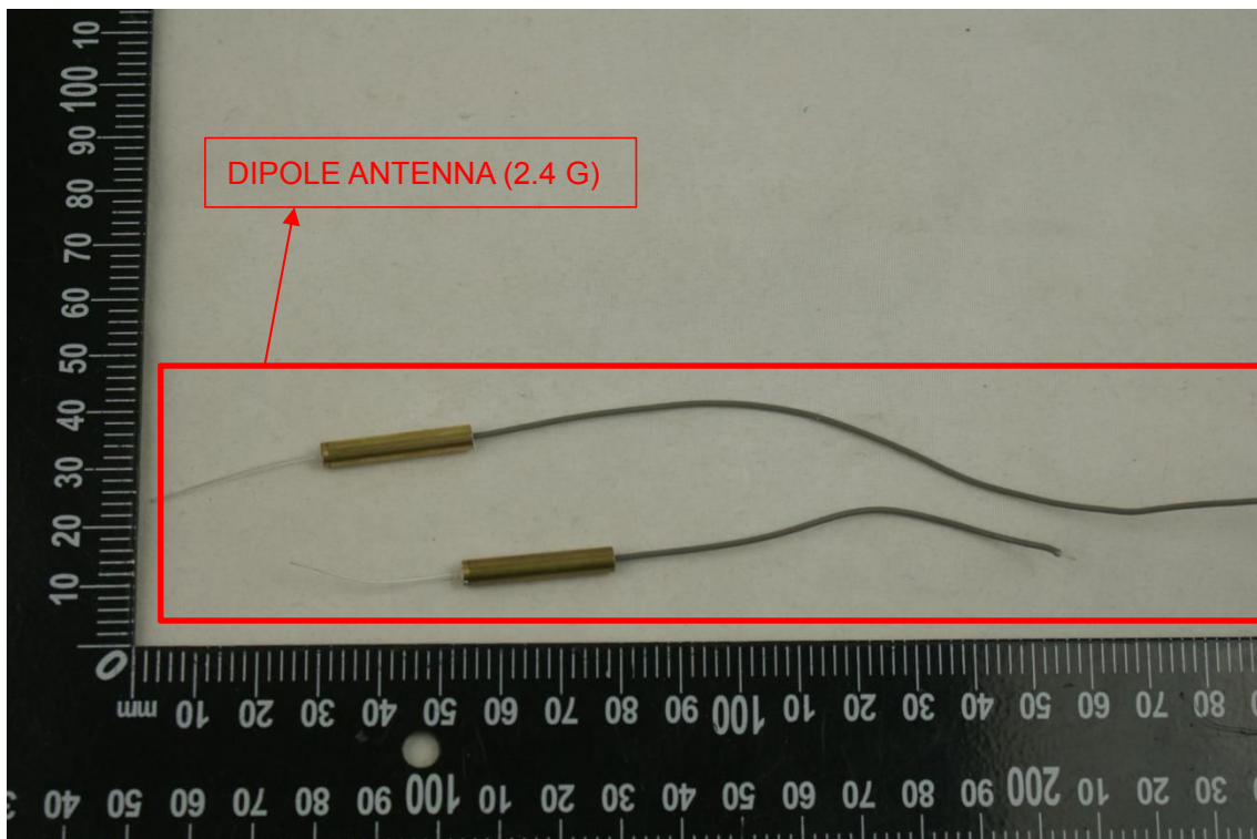
EUT PHOTO 4
