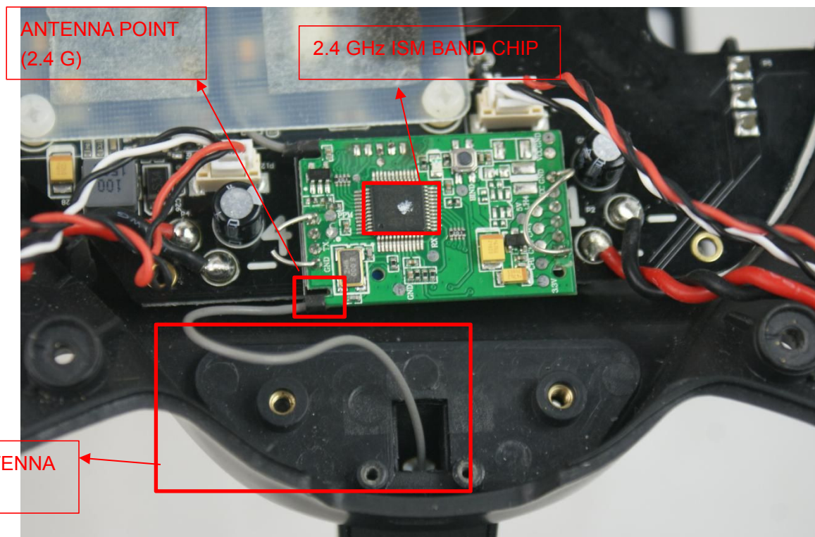
EUT PHOTO 2
