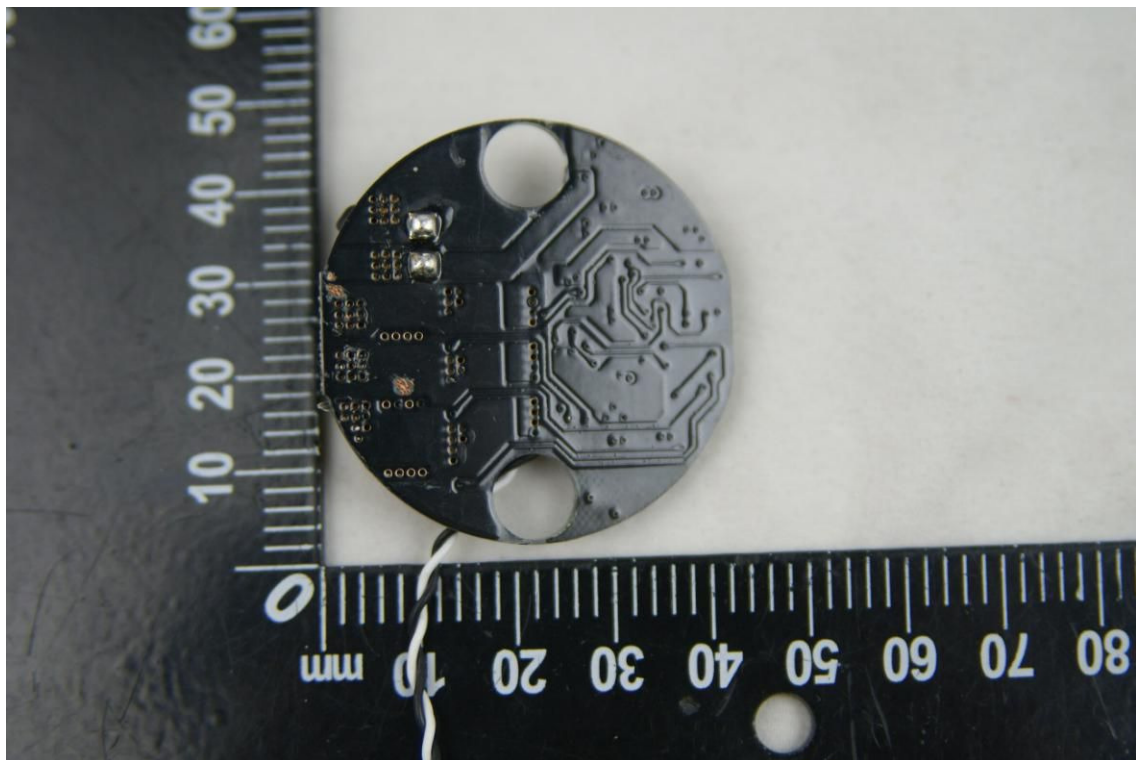
EUT PHOTO 18
