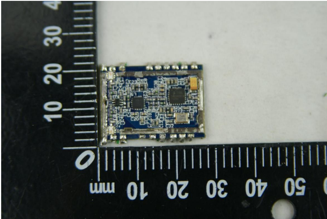
EUT PHOTO 31
