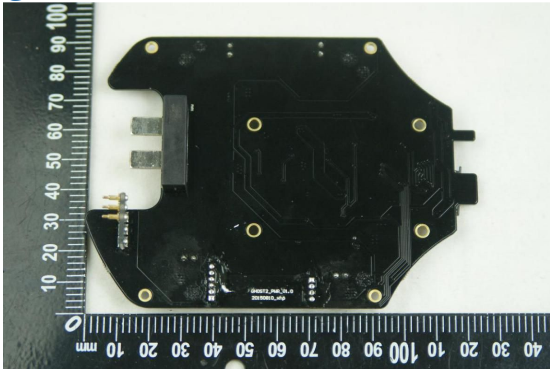
EUT PHOTO 25
