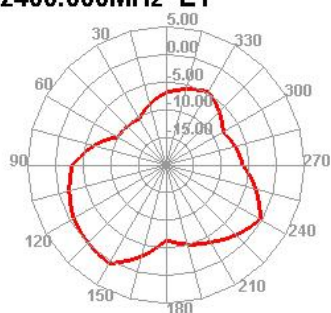
2400.000MHz E1
