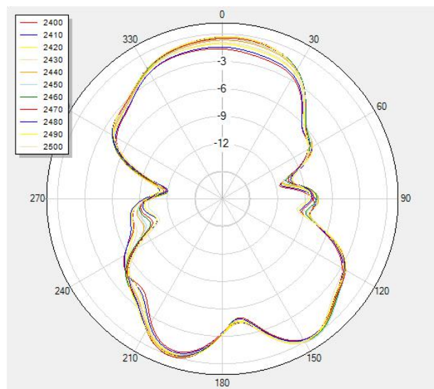
V Phi=90
