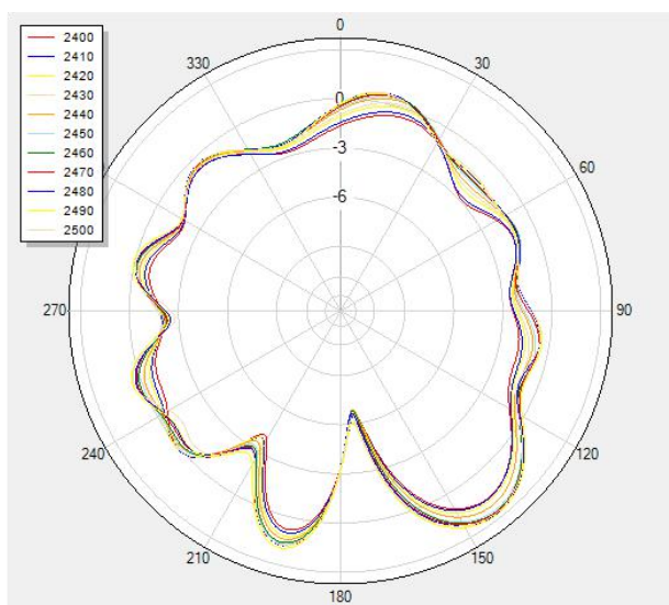
V Phi=0
