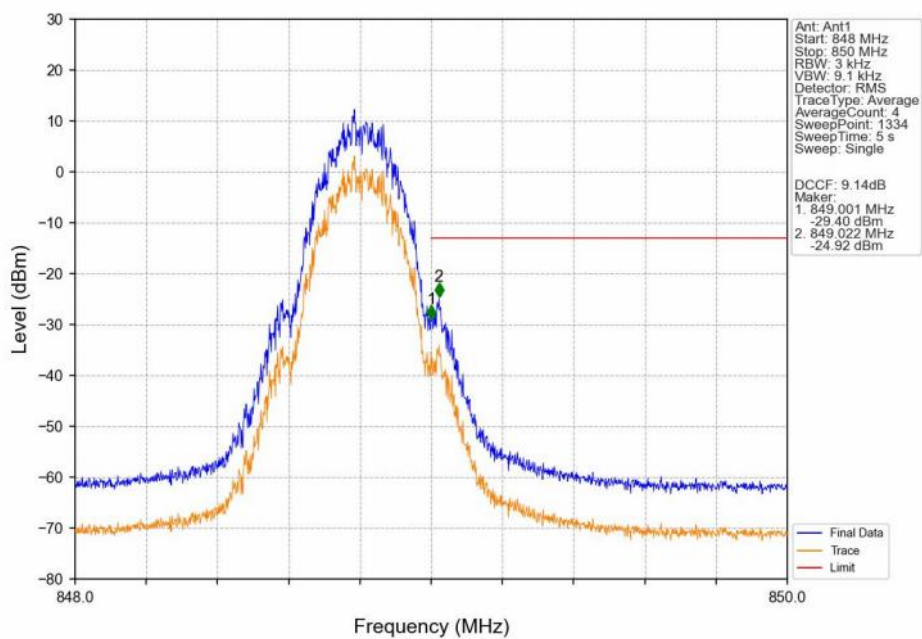
GSM850_GSM_HCH_848.8MHz_GSM_NTNV
