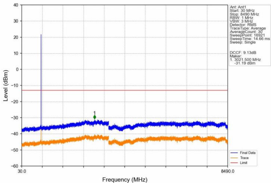
GSM850_GSM_MCH_836.6MHz_GSM_NTNV
