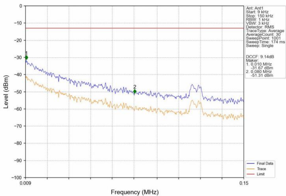
GSM850_GSM_MCH_836.6MHz_GSM_NTNV
