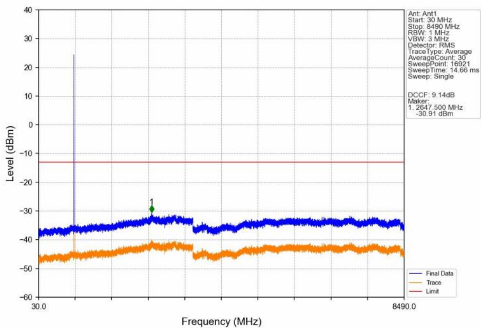
GSM850_GSM_HCH_848.8MHz_GSM_NTNV
