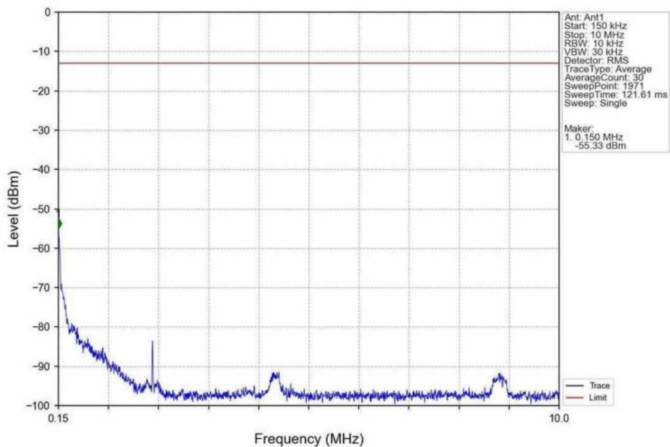
Band25_10MHz_QPSK_LCH_1855MHz_RB_1_0_NTNV
