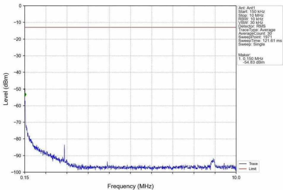
Band25_20MHz_QPSK_HCH_1905MHz_RB_1_0_NTNV
