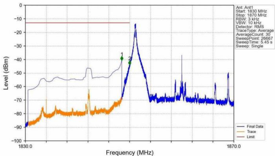
Band25_20MHz_QPSK_LCH_1860MHz_RB_1_0_NTNV
