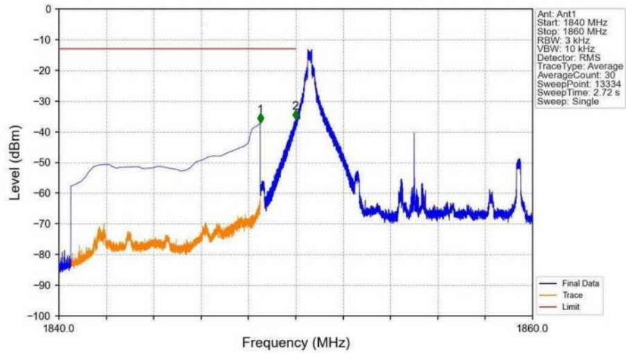
Band25_10MHz_QPSK_LCH_1855MHz_RB_1_0_NTNV
