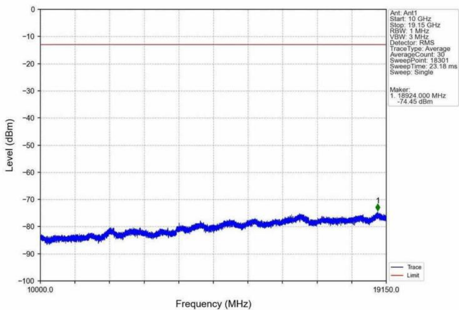
Band25_10MHz_QPSK_LCH_1855MHz_RB_1_0_NTNV
