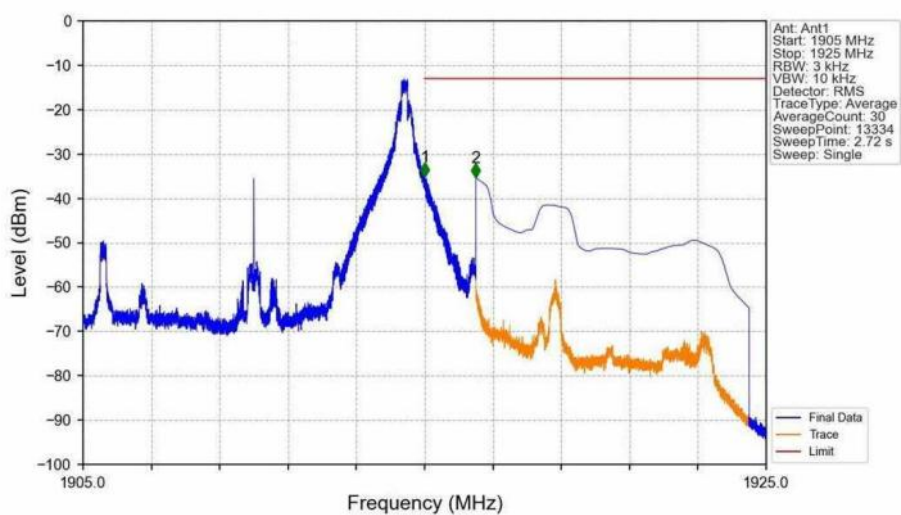
Band25_10MHz_QPSK_HCH_1910MHz_RB_1_49_NTNV
