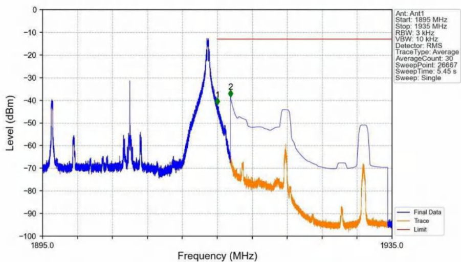
Band25_20MHz_QPSK_HCH_1905MHz_RB_1_99_NTNV
