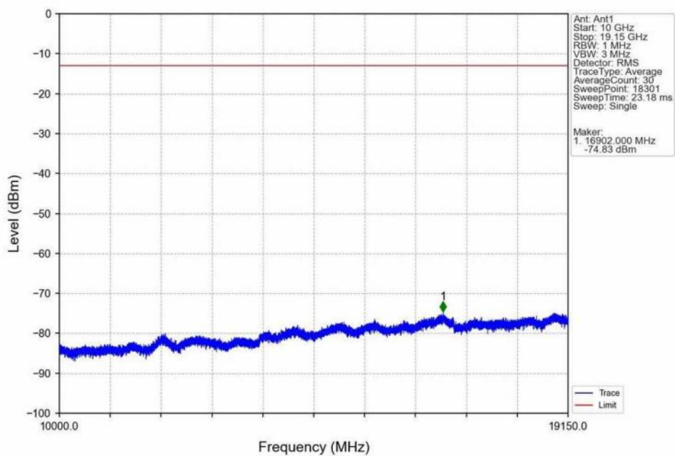
Band25_20MHz_QPSK_LCH_1860MHz_RB_1_0_NTNV
