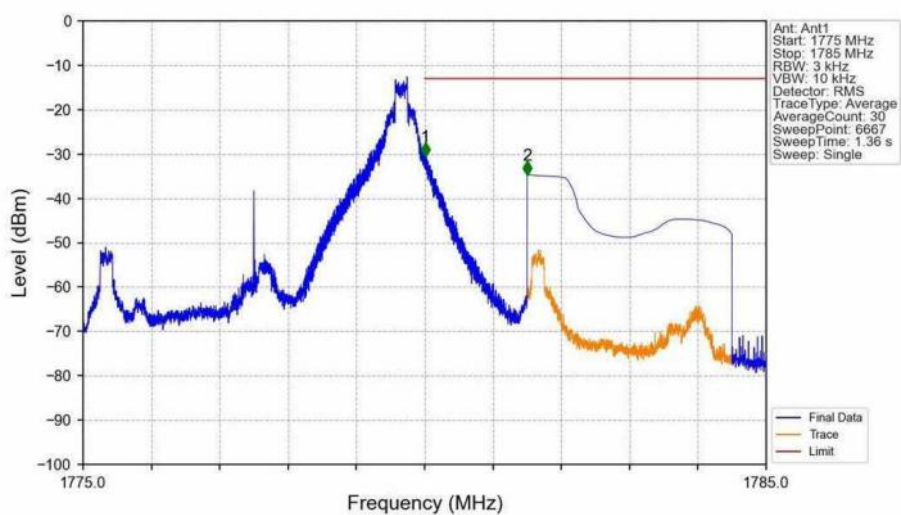
Band66_5MHz_QPSK_HCH_1777.5MHz_RB_1_24_NTNV
