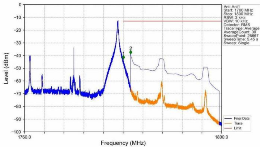
Band66_20MHz_16QAM_HCH_1770MHz_RB_1_99_NTNV
