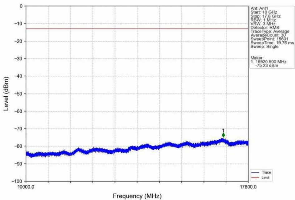
Band66_20MHz_QPSK_LCH_1720MHz_RB_1_0_NTNV
