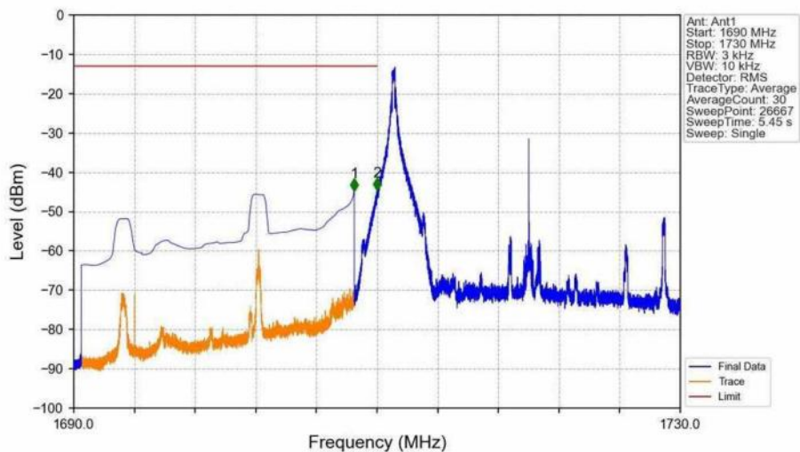
Band66_20MHz_QPSK_LCH_1720MHz_RB_1_0_NTNV
