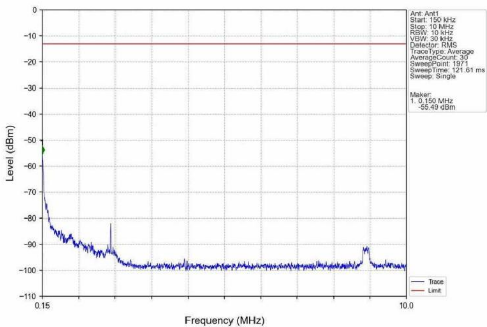
Band66_20MHz_QPSK_HCH_1770MHz_RB_1_0_NTNV
