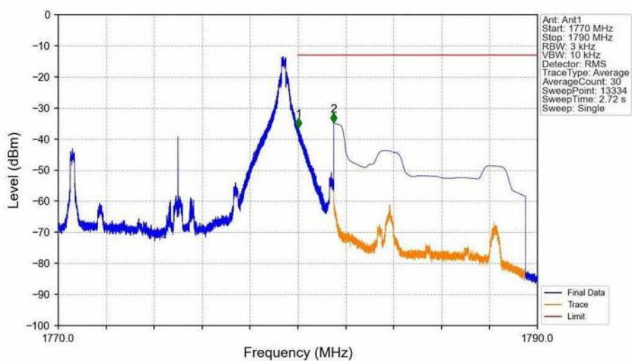
Band66_10MHz_QPSK_HCH_1775MHz_RB_1_49_NTNV
