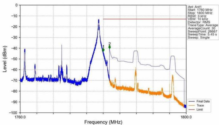
Band66_20MHz_QPSK_HCH_1770MHz_RB_1_99_NTNV
