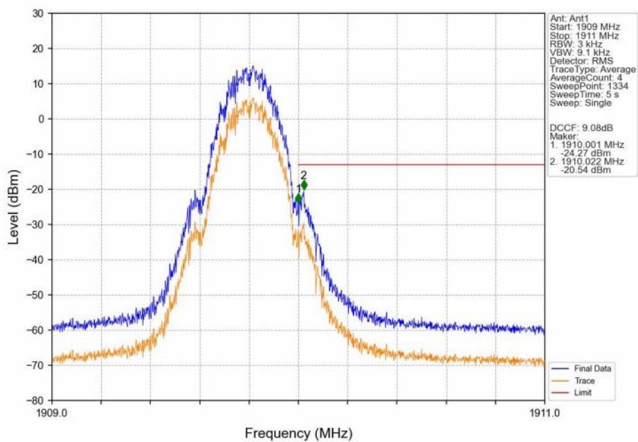
PCS1900_GSM_HCH_1909.8MHz_GSM_NTNV
