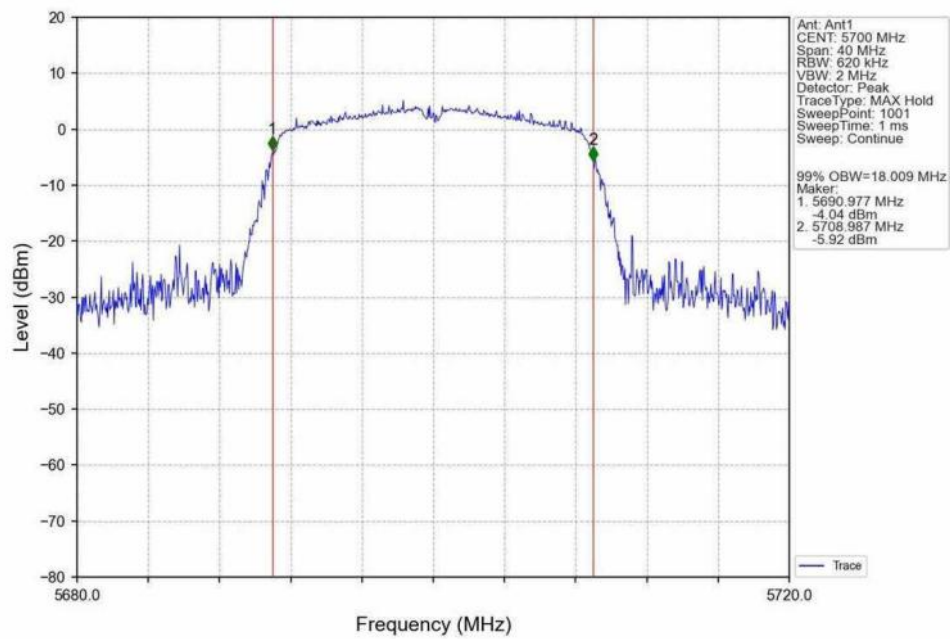
802.11ac(VHT20)_HCH_5700MHz_Ant1_NTNV
