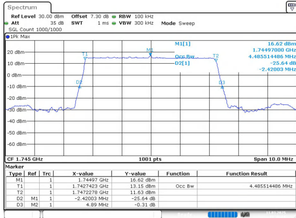
n66 SCS=15kHz DFT_BPSK BW=5MHz Channel=349000 RB=25@0
