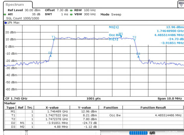
n66 SCS=15kHz CP_QPSK BW=5MHz Channel=349000 RB=25@0
